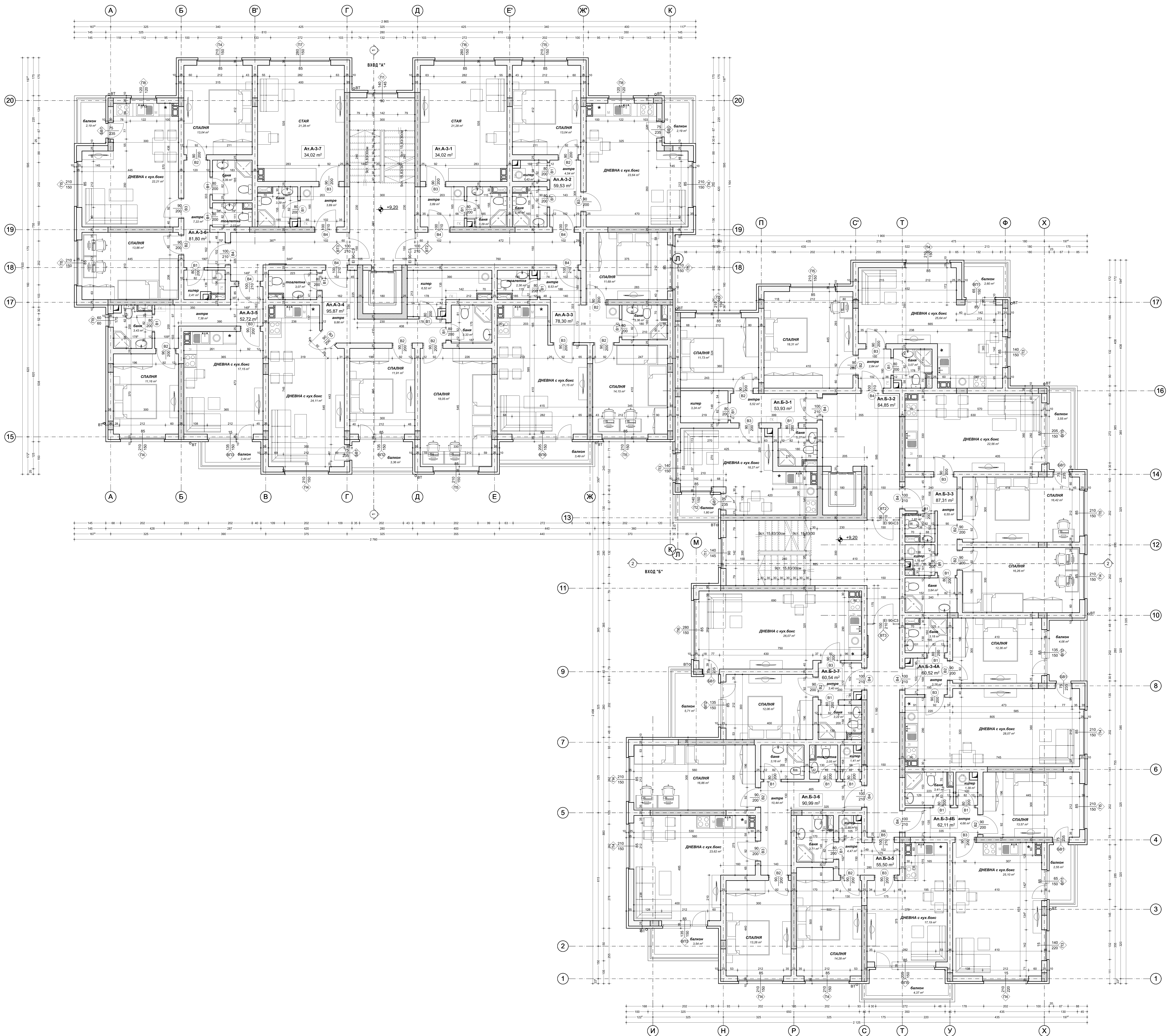
РАЗПРЕДЕЛЕНИЕ III ЖИЛИЩЕН ЕТАЖ
