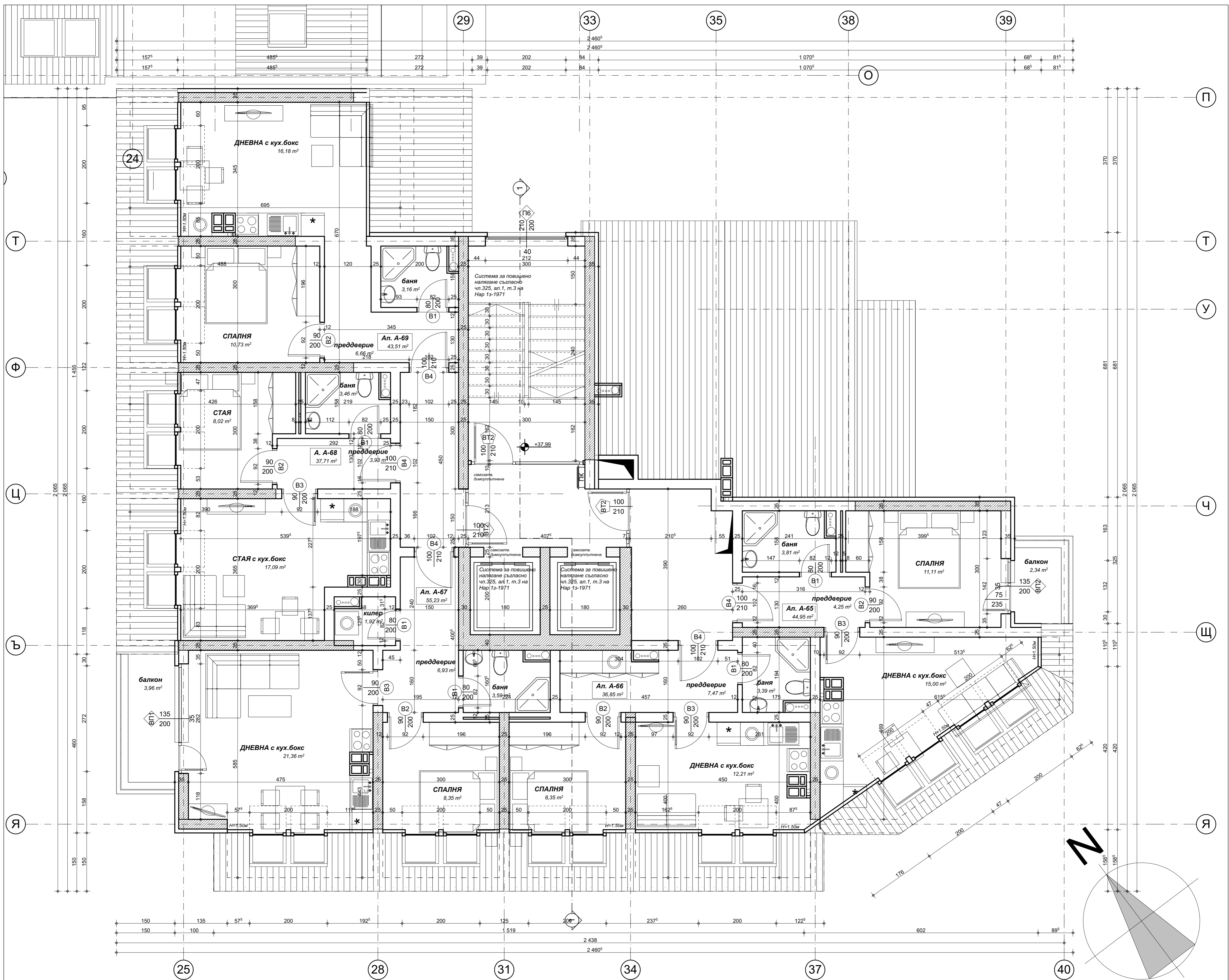
РАЗПРЕДЕЛЕНИЕ I ПОДПОКРИВЕН ЕТАЖ
