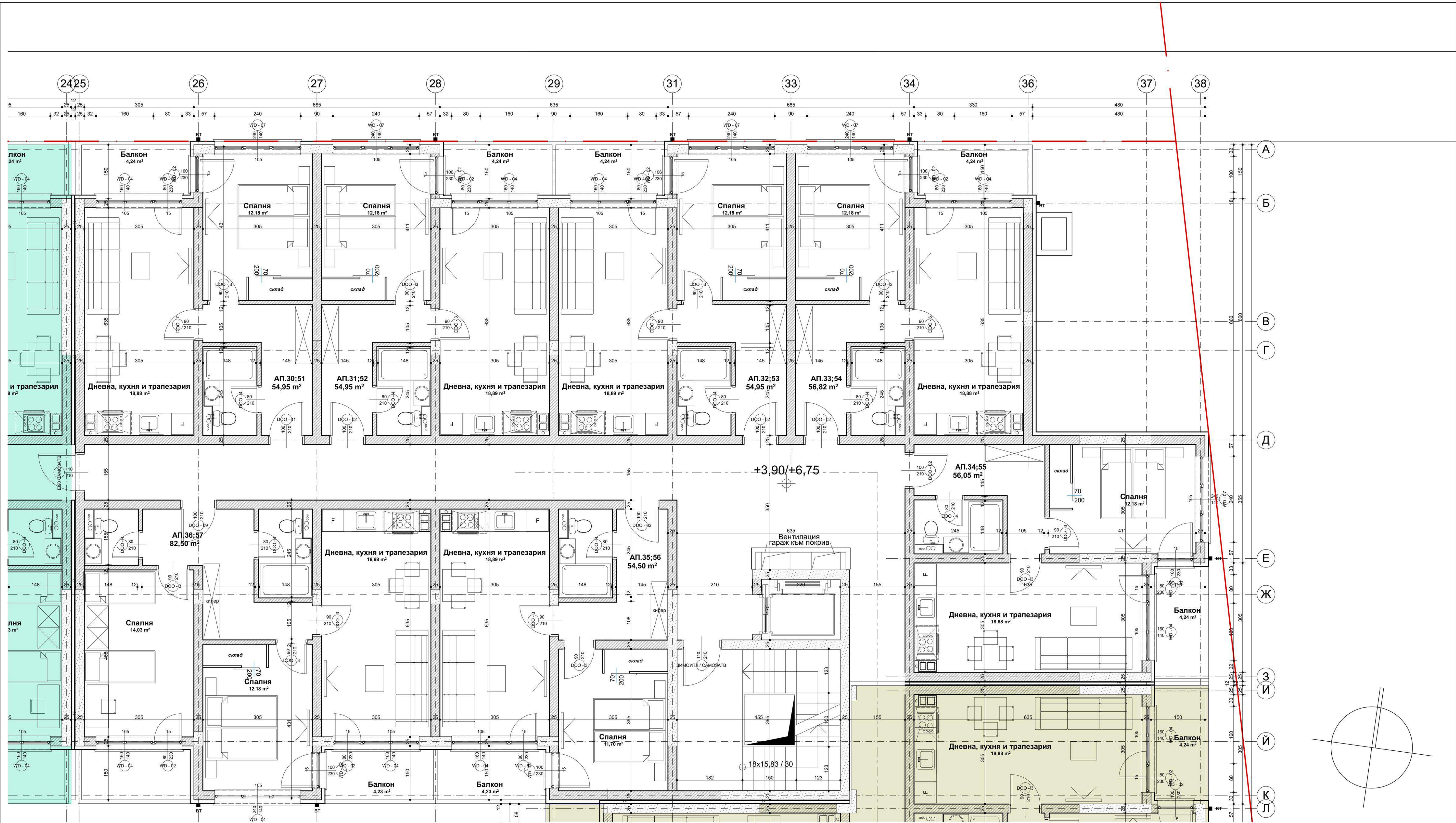
РАЗПРЕДЕЛЕНИЕ II, III ЕТАЖ
