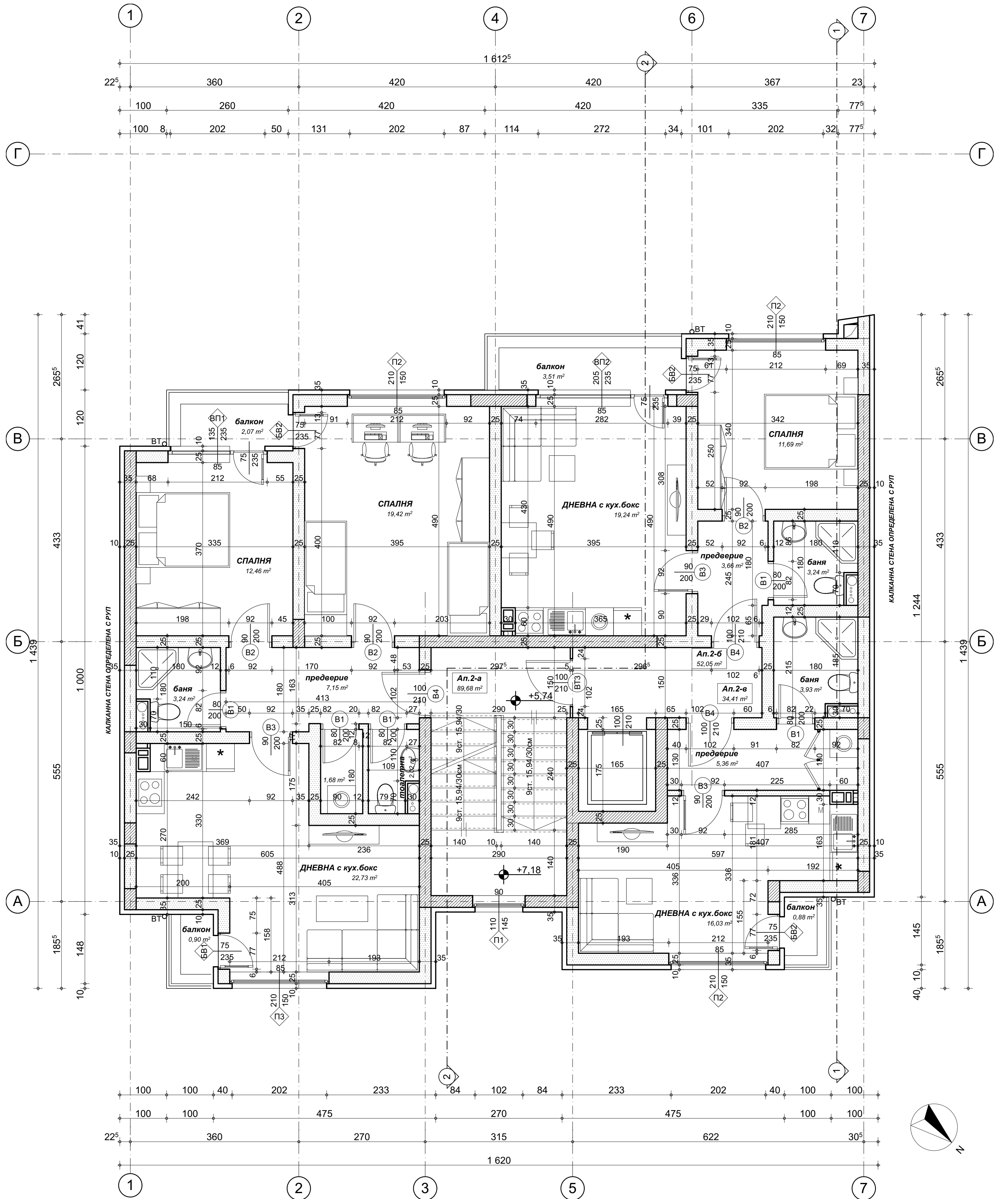
РАЗПРЕДЕЛЕНИЕ II ЖИЛИЩЕН ЕТАЖ М1:50
