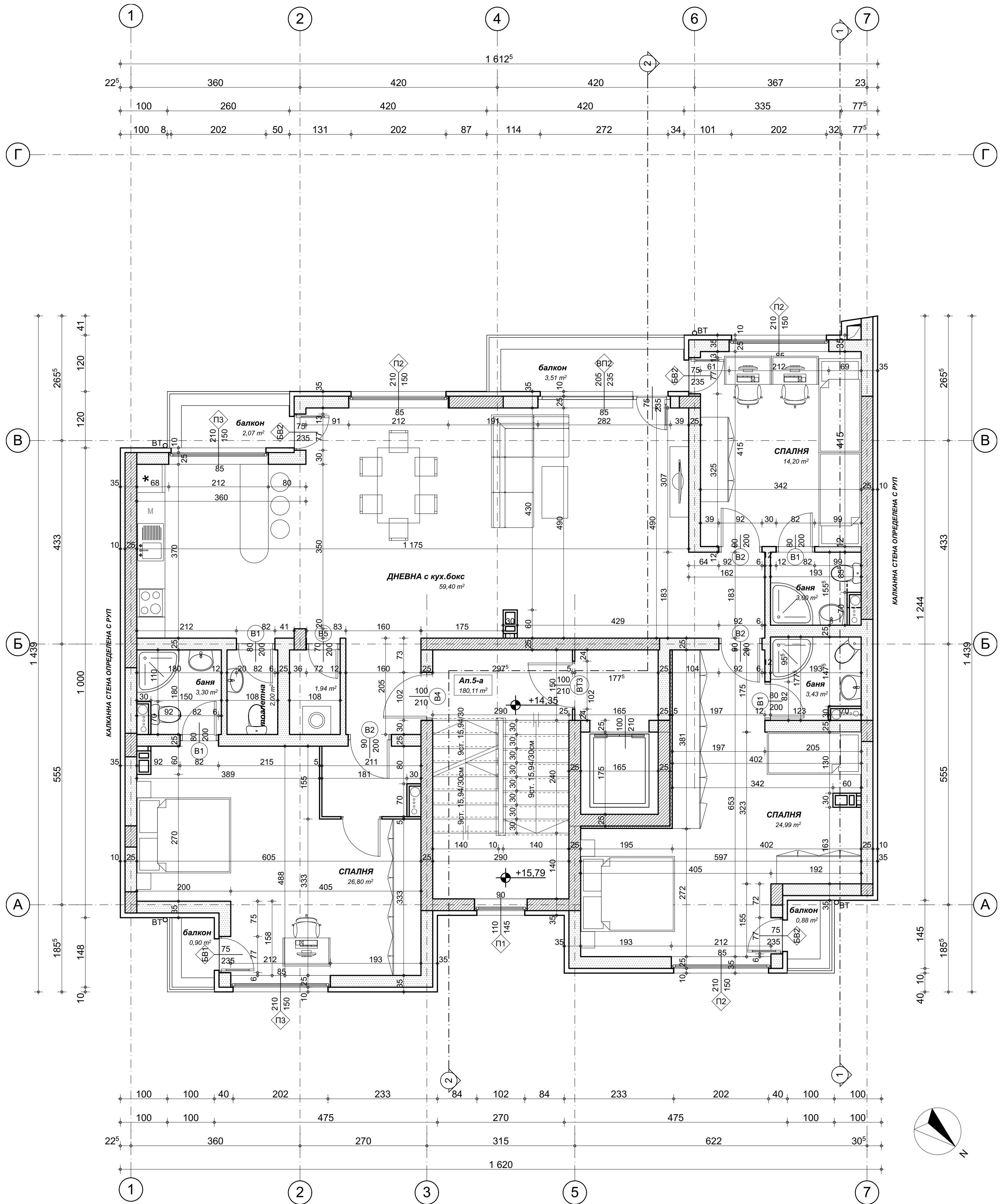
РАЗПРЕДЕЛЕНИЕ V ЖИЛИЩЕН ЕТАЖ М1:50
