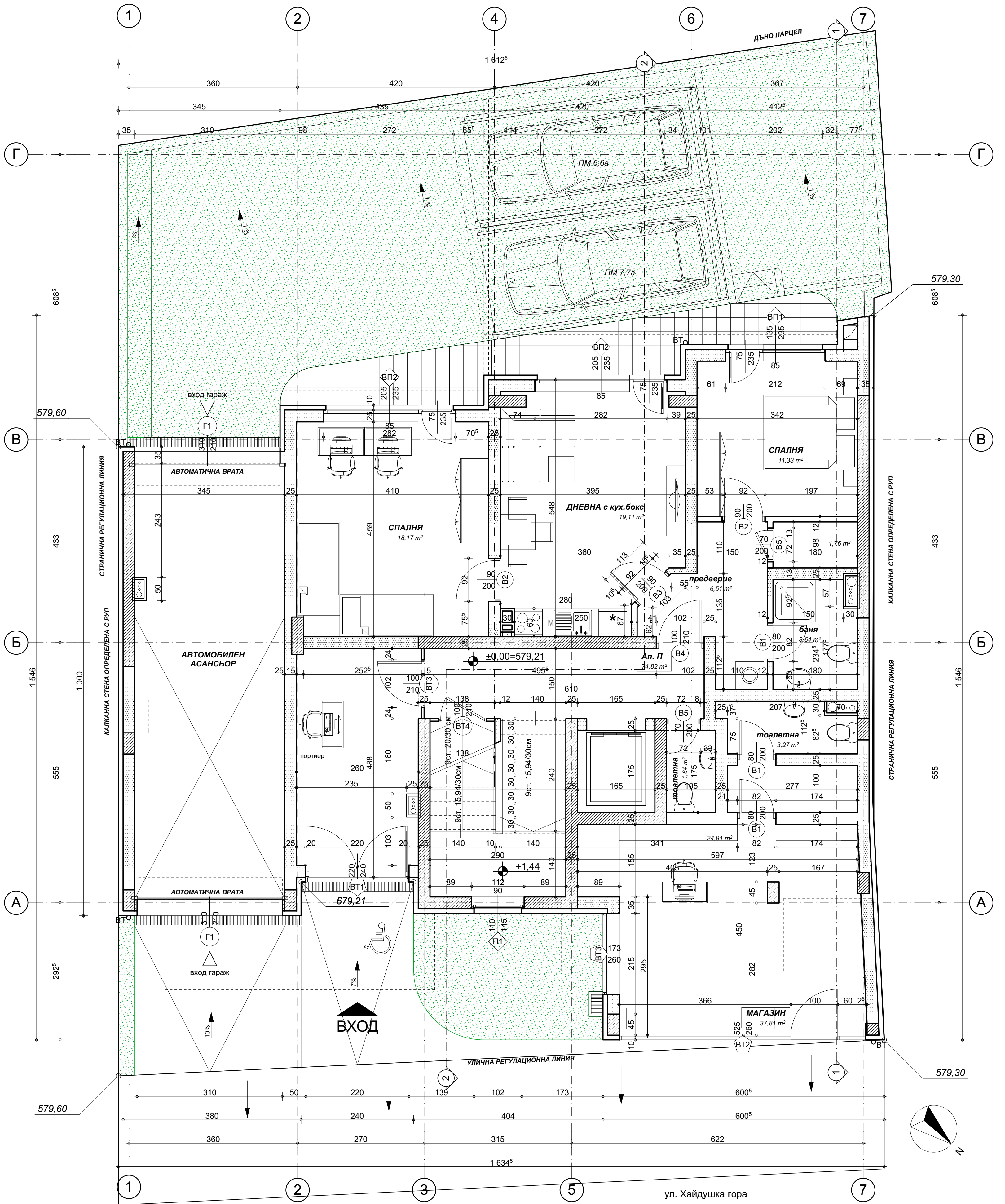
РАЗПРЕДЕЛЕНИЕ ПАРТЕР М1:50
