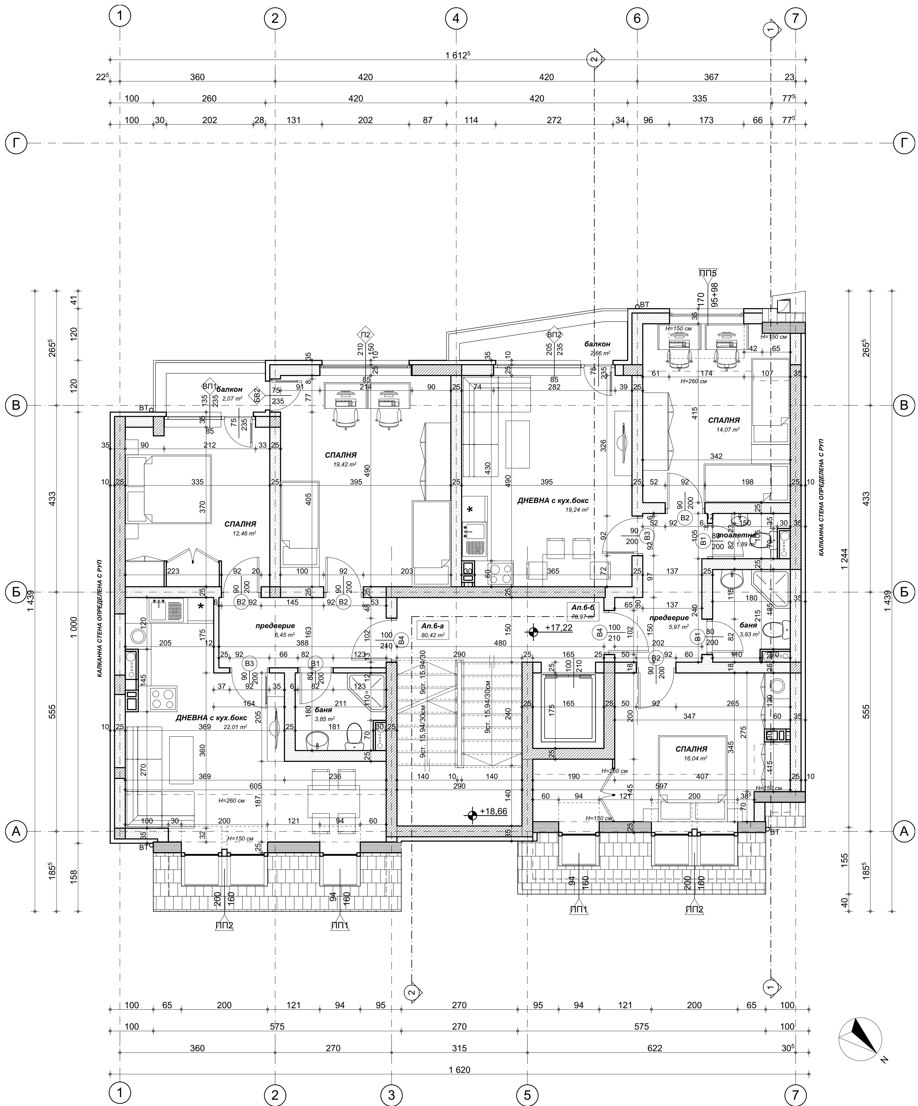
РАЗПРЕДЕЛЕНИЕ VI ЖИЛИЩЕН ЕТАЖ М1:50
