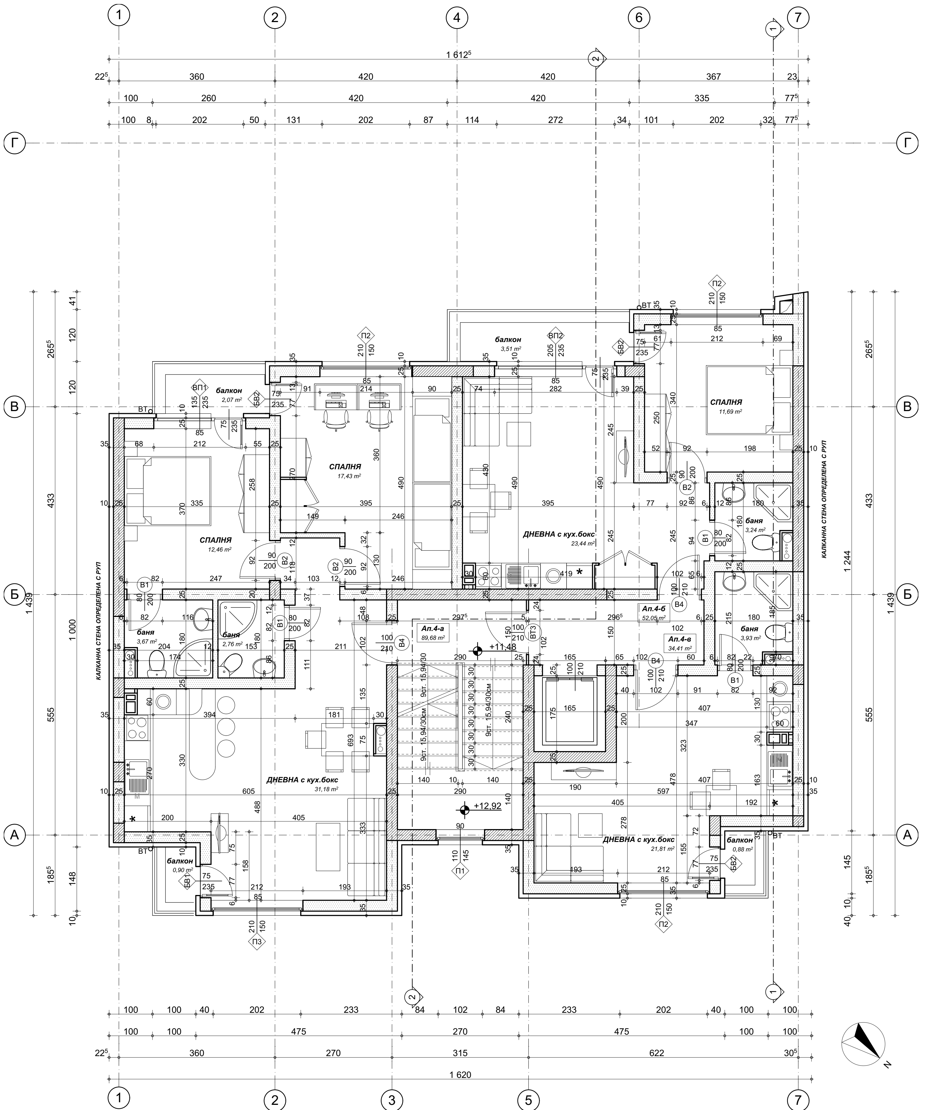
РАЗПРЕДЕЛЕНИЕ IV ЖИЛИЩЕН ЕТАЖ М1:50
