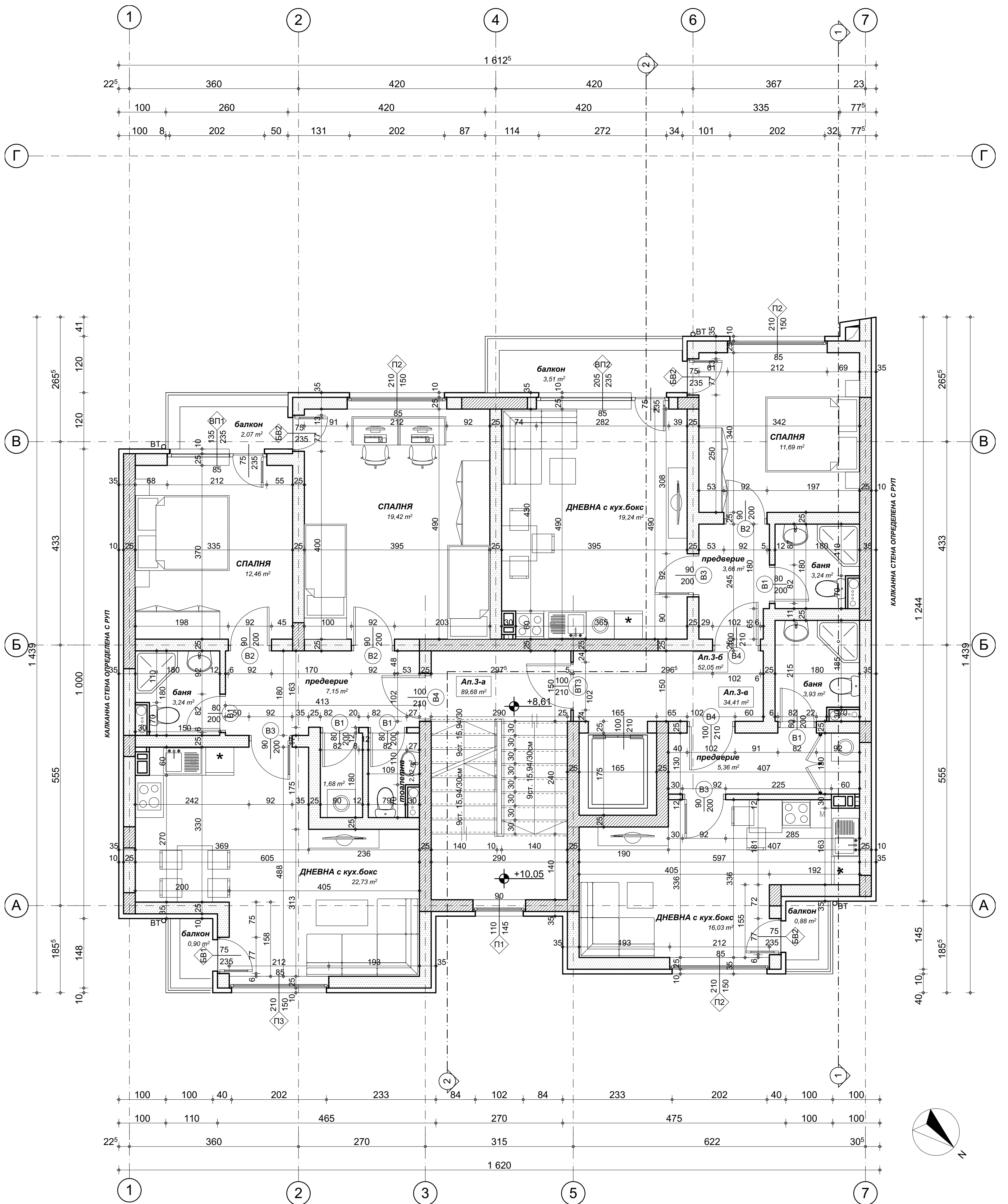
РАЗПРЕДЕЛЕНИЕ III ЖИЛИЩЕН ЕТАЖ М1:50
