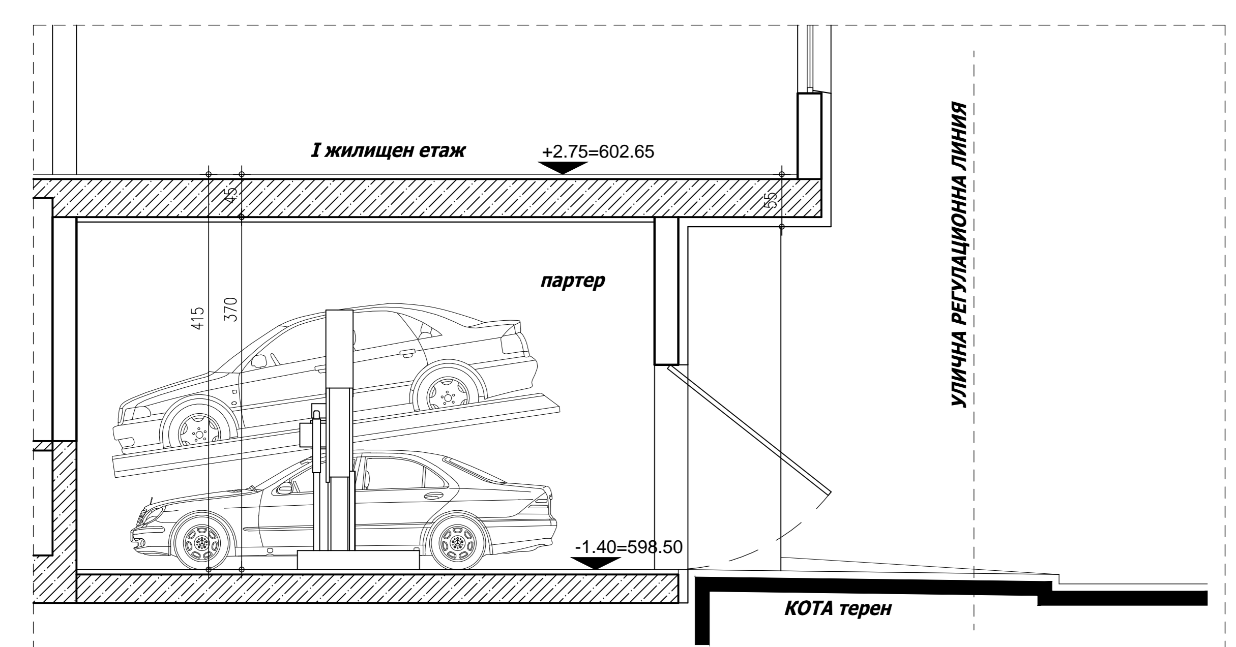
ВЕРТИКАЛЕН РАЗРЕЗ
