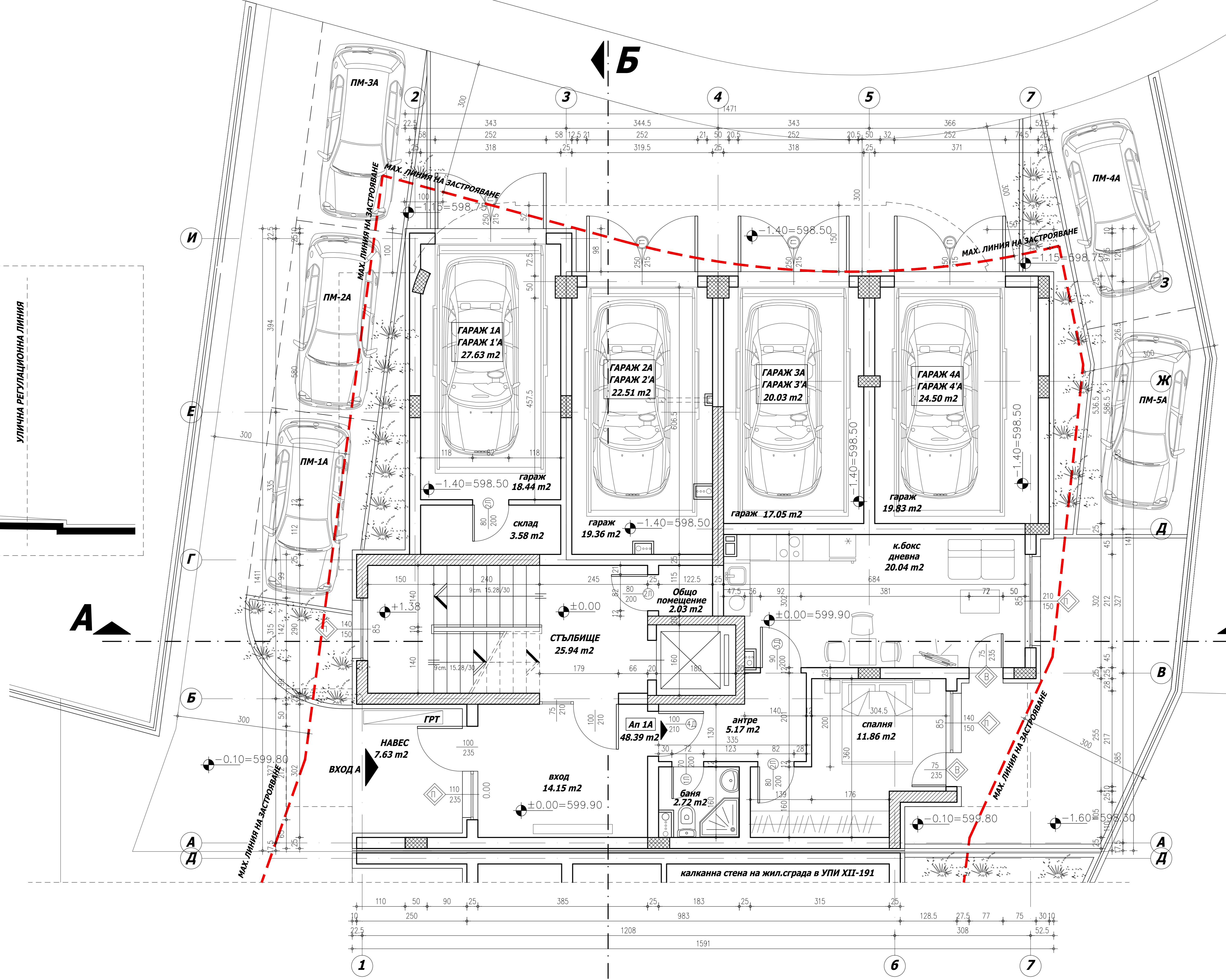
РАЗПРЕДЕЛЕНИЕ ПАРТЕР М 1:50
