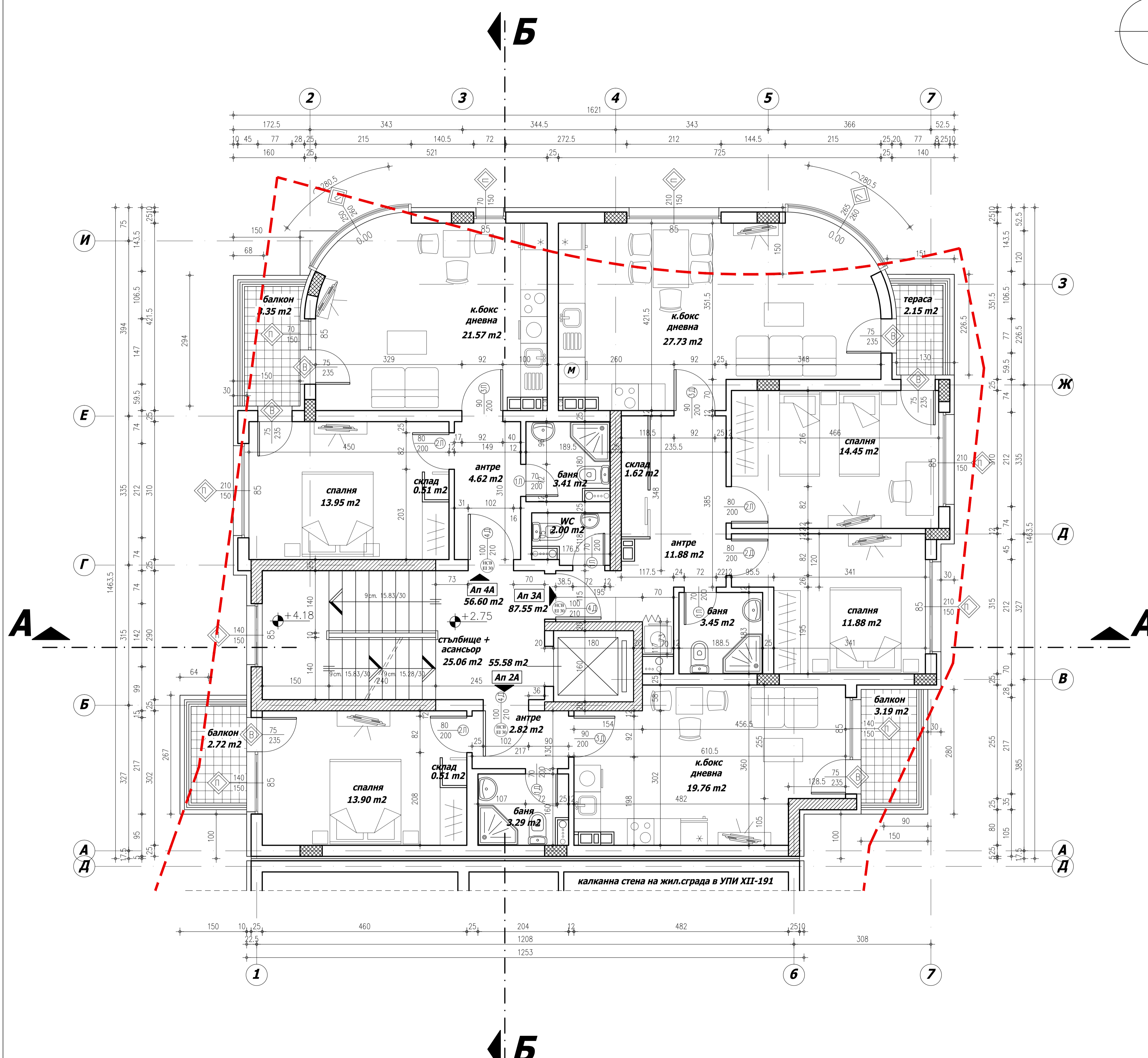
РАЗПРЕДЕЛЕНИЕ I ЕТАЖ М 1:50
