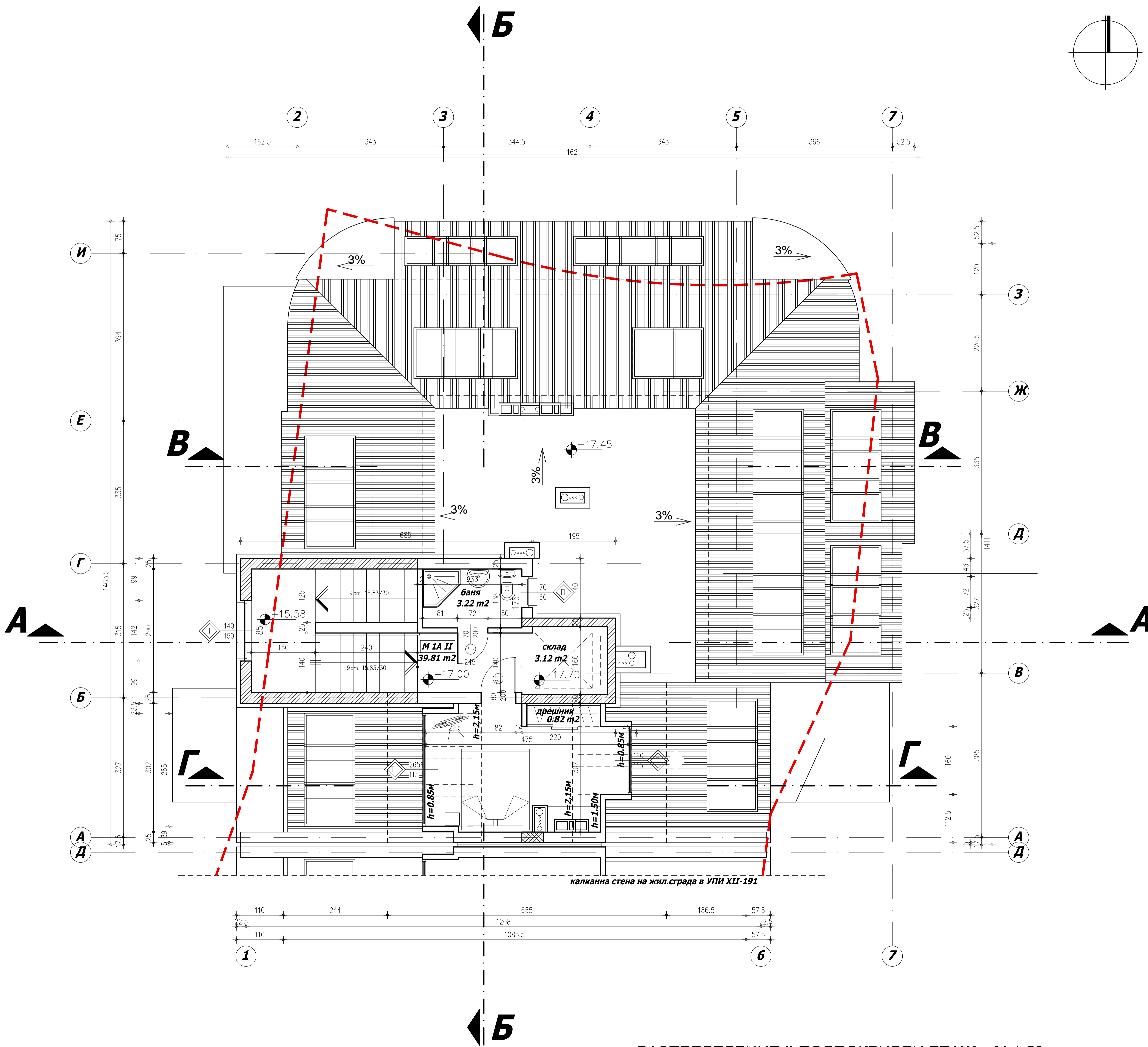
РАЗПРЕДЕЛЕНИЕ II ПОДПОКРИВЕН ЕТАЖ М 1:50
