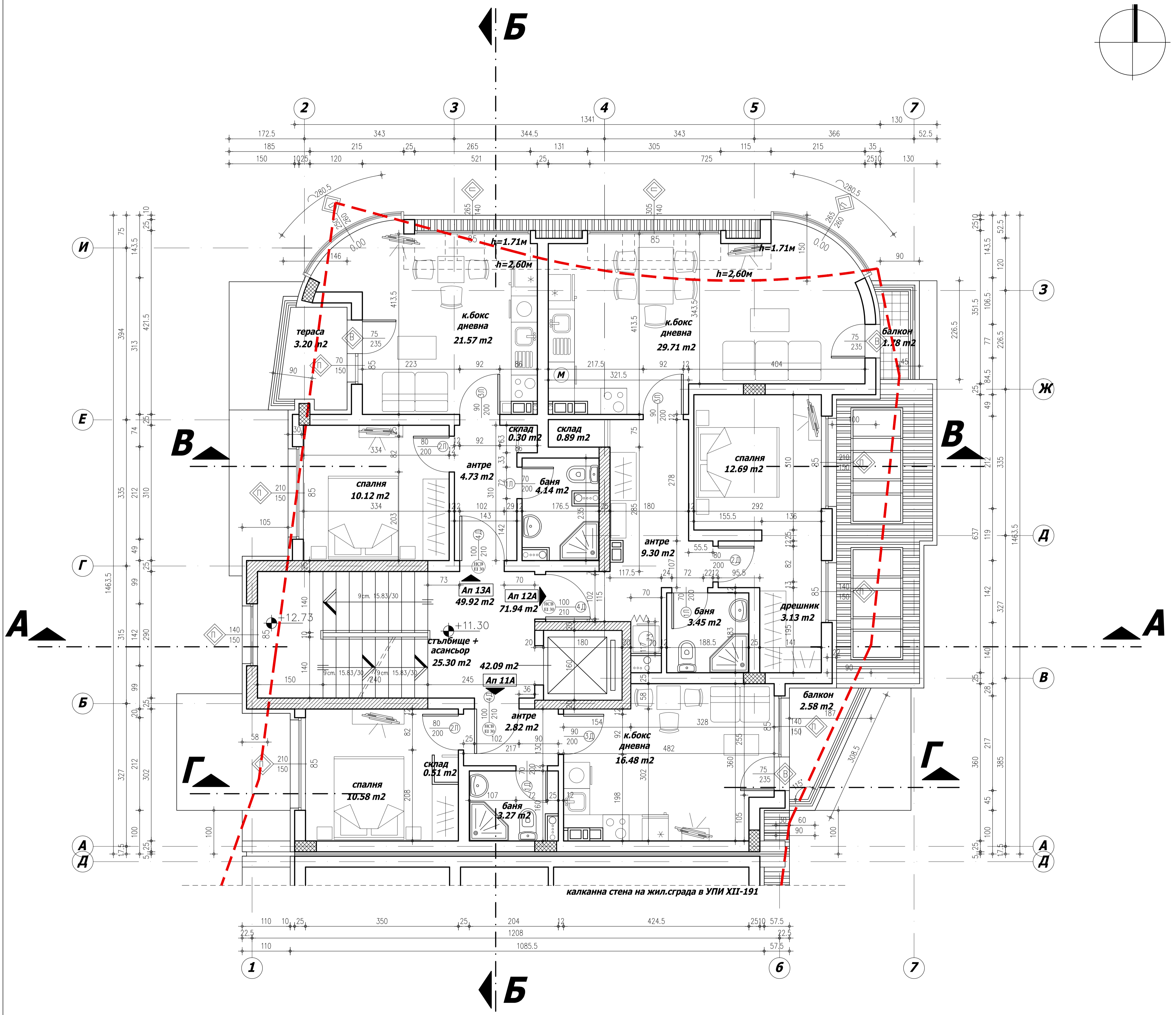
РАЗПРЕДЕЛЕНИЕ IV ЕТАЖ М 1:50
