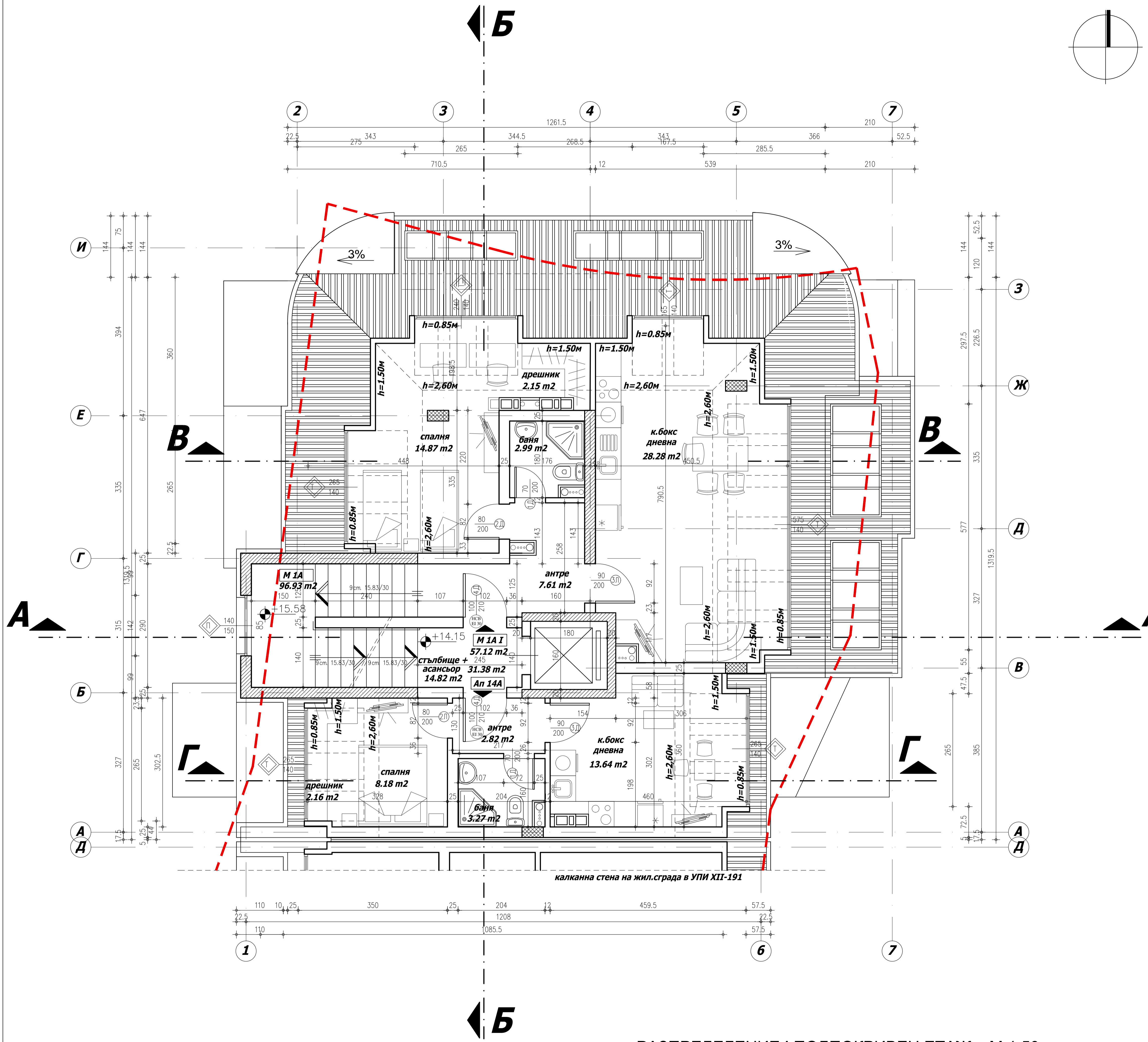
РАЗПРЕДЕЛЕНИЕ I ПОДПОКРИВЕН ЕТАЖ М 1:50
