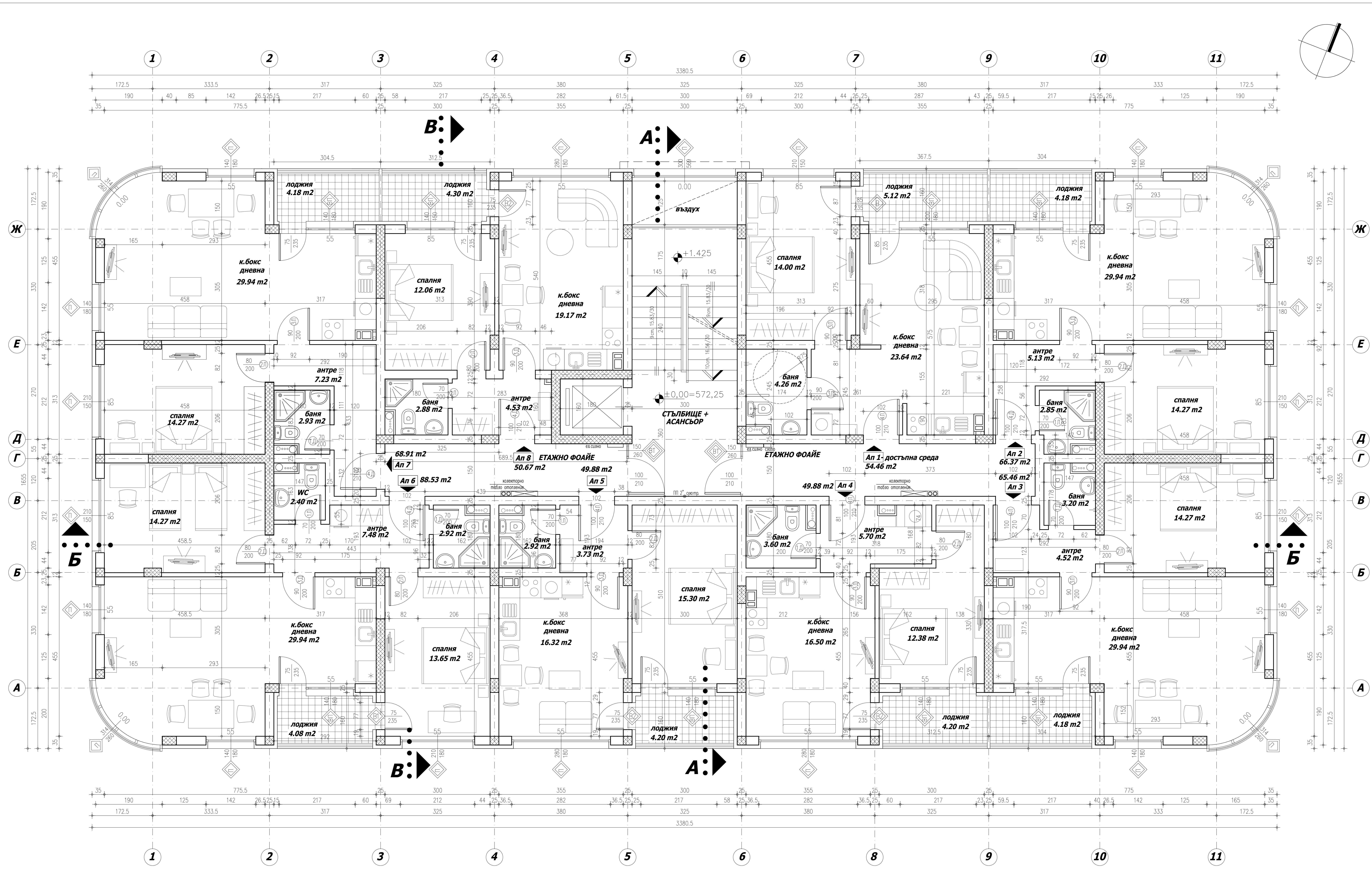
РАЗПРЕДЕЛЕНИЕ ПЪРВИ ЕТАЖ М 1:50
