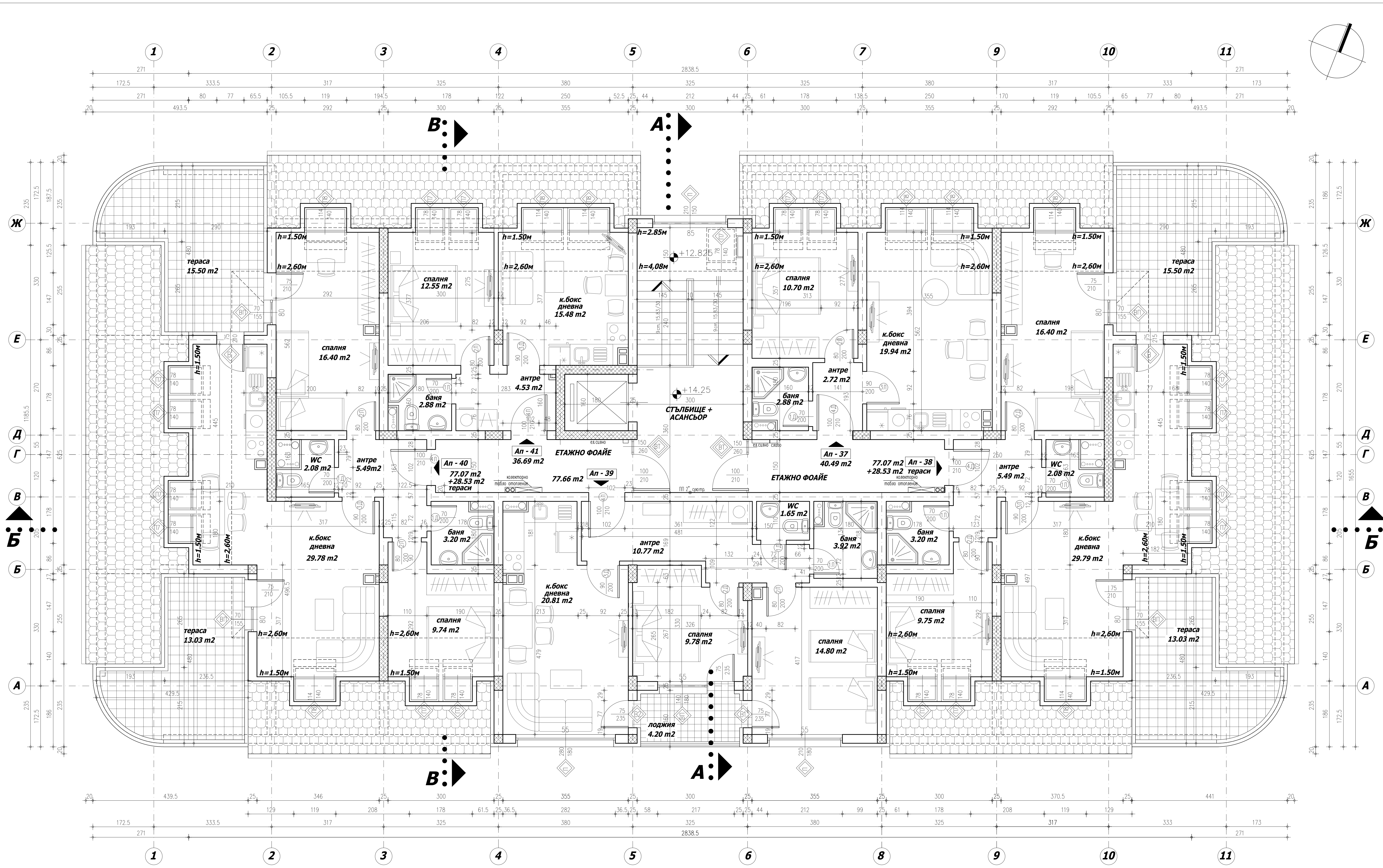
РАЗПРЕДЕЛЕНИЕ II ПОДПОКРИВЕН ЕТАЖ М 1:50
