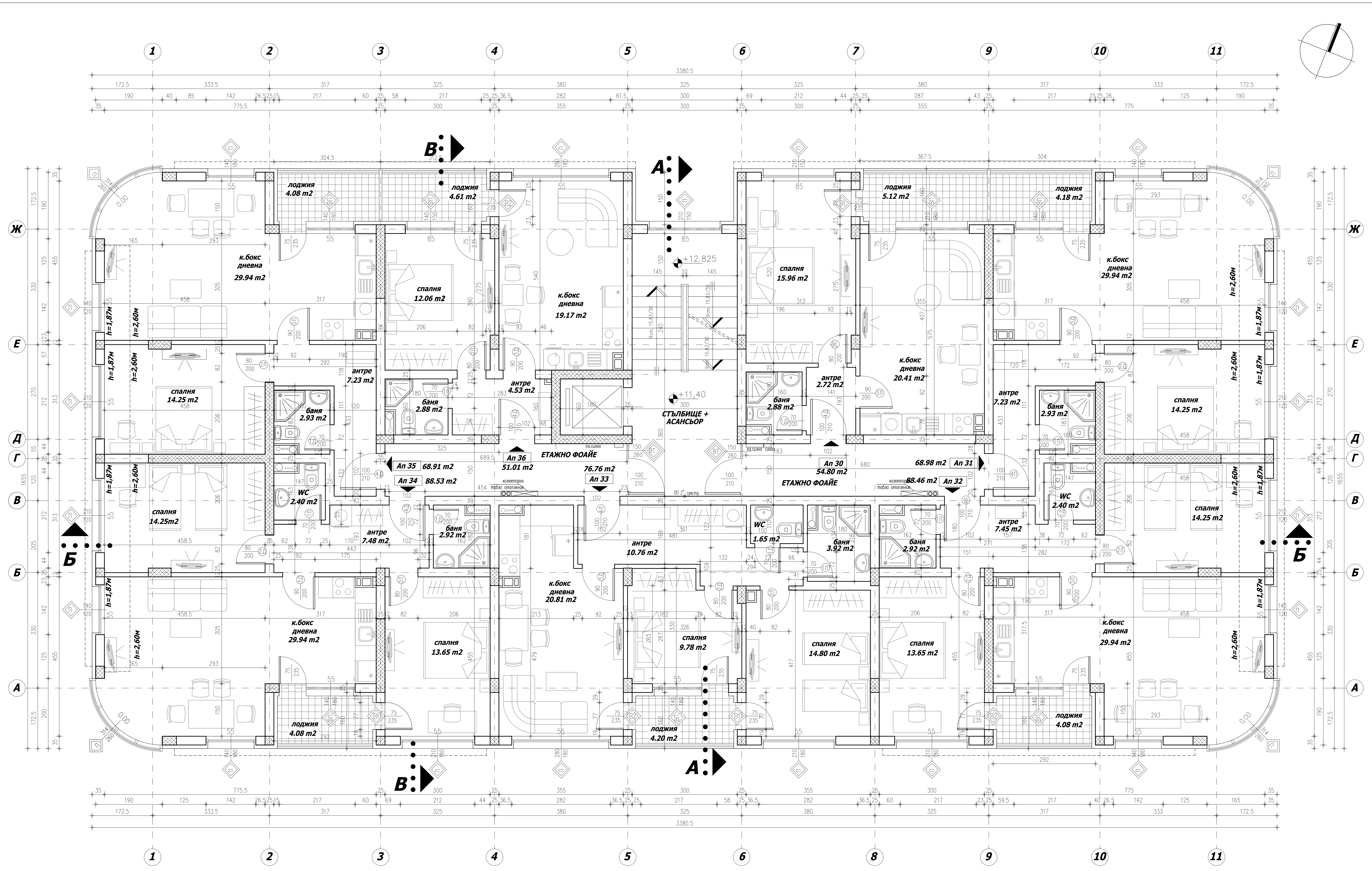
РАЗПРЕДЕЛЕНИЕ I ПОДПОКРИВЕН ЕТАЖ М 1:50
