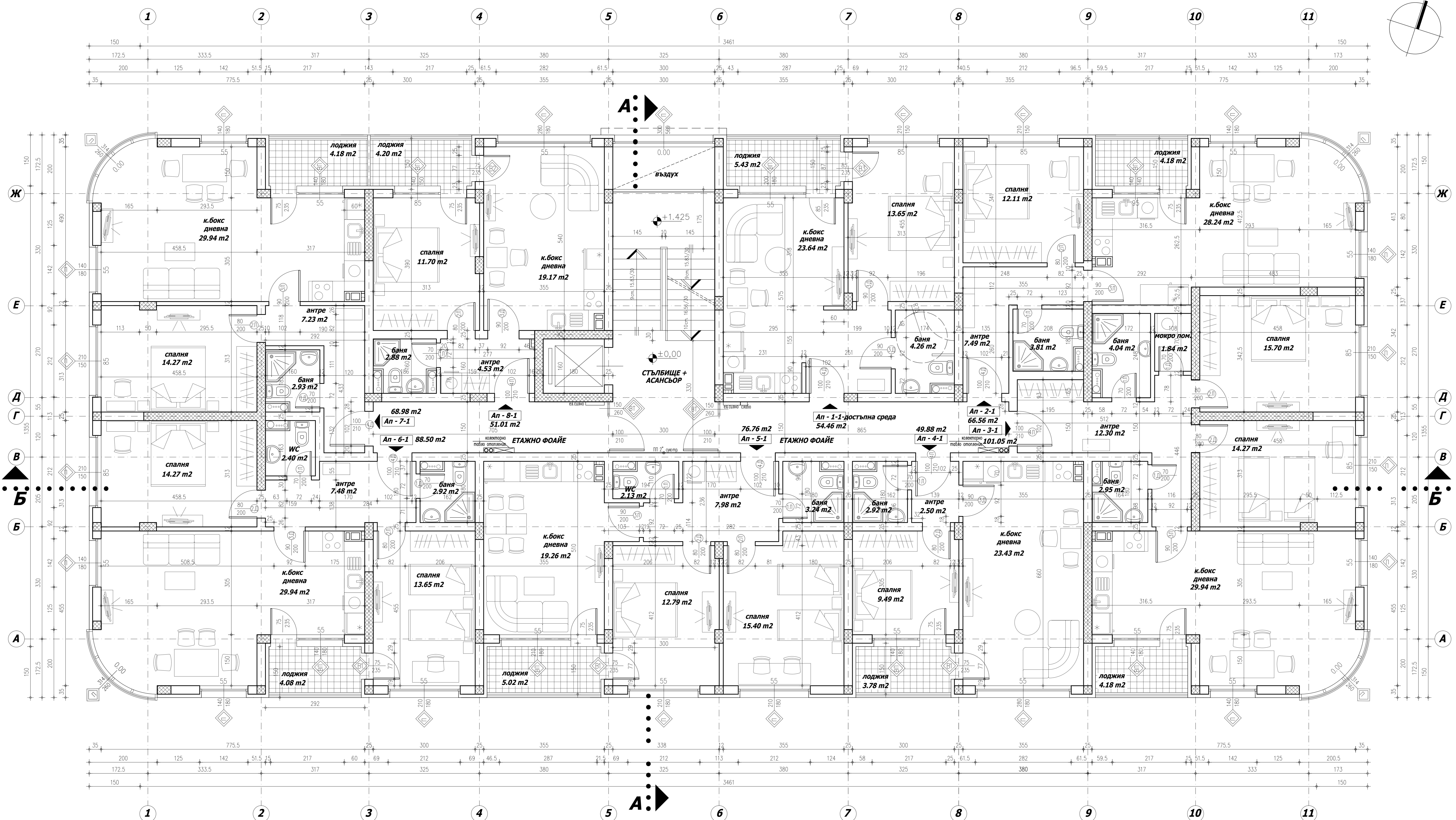
РАЗПРЕДЕЛЕНИЕ ПЪРВИ ЕТАЖ М 1:50
