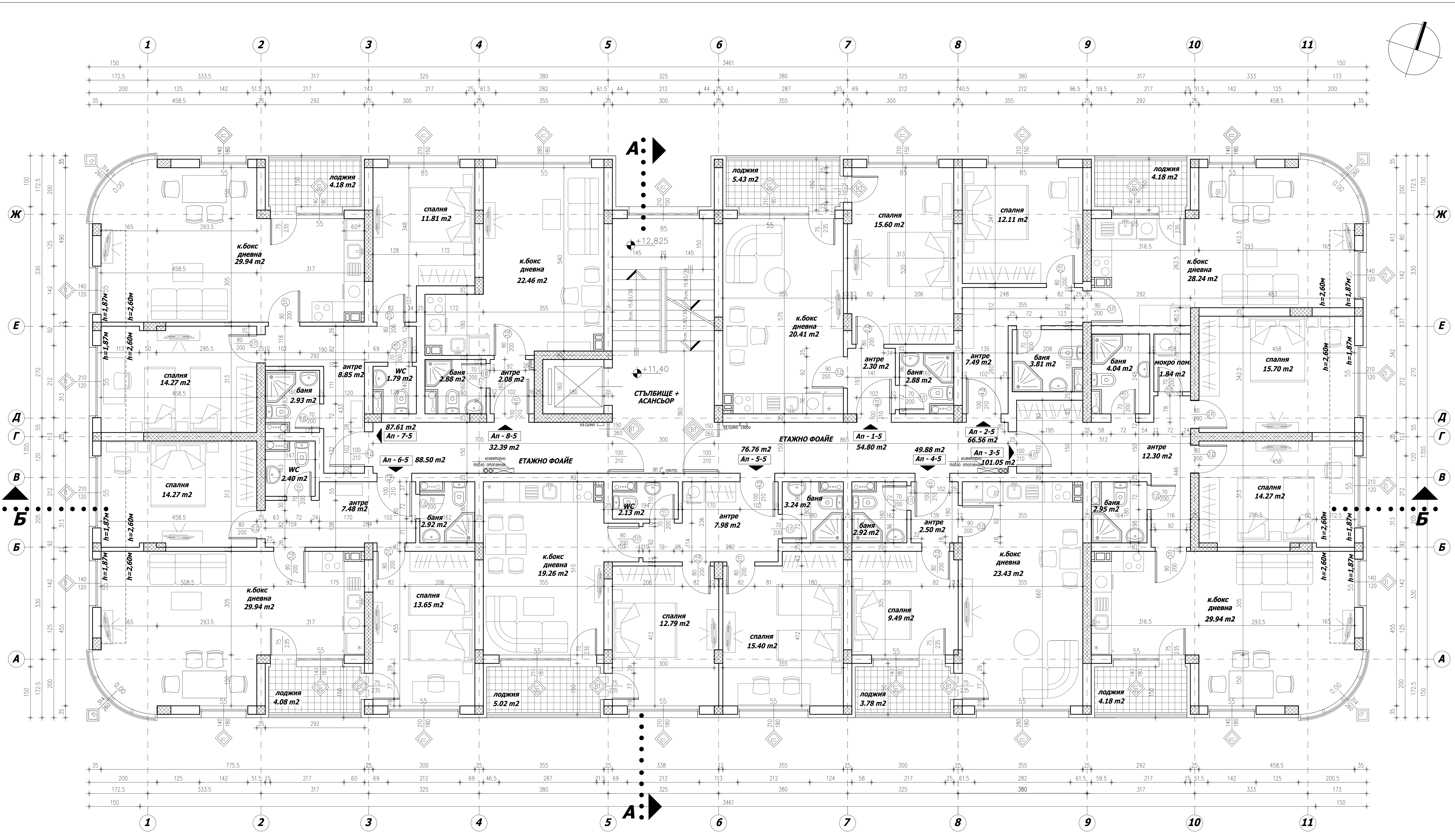
РАЗПРЕДЕЛЕНИЕ I ПОДПОКРИВЕН ЕТАЖ М 1:50
