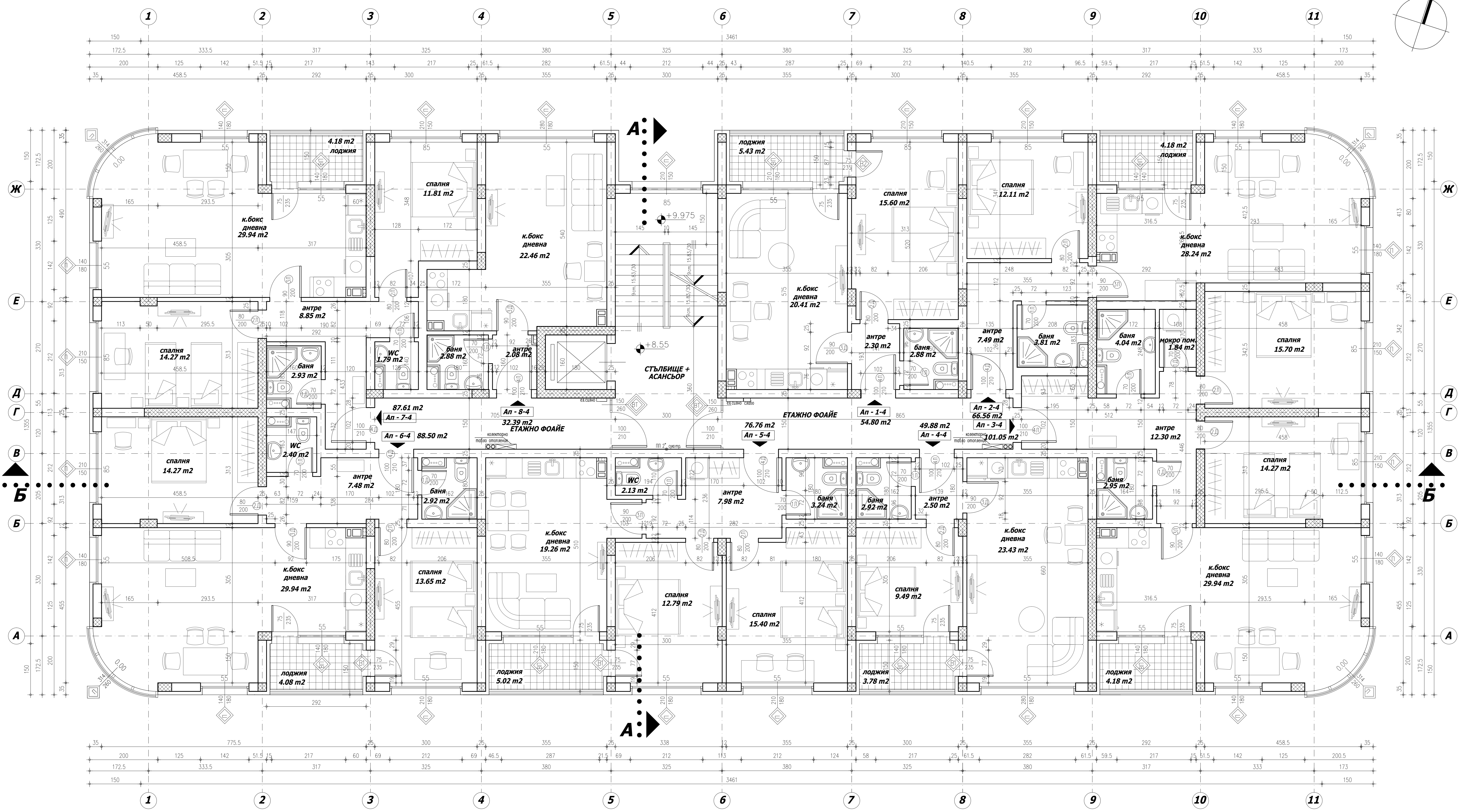
РАЗПРЕДЕЛЕНИЕ IV ЕТАЖ М 1:50
