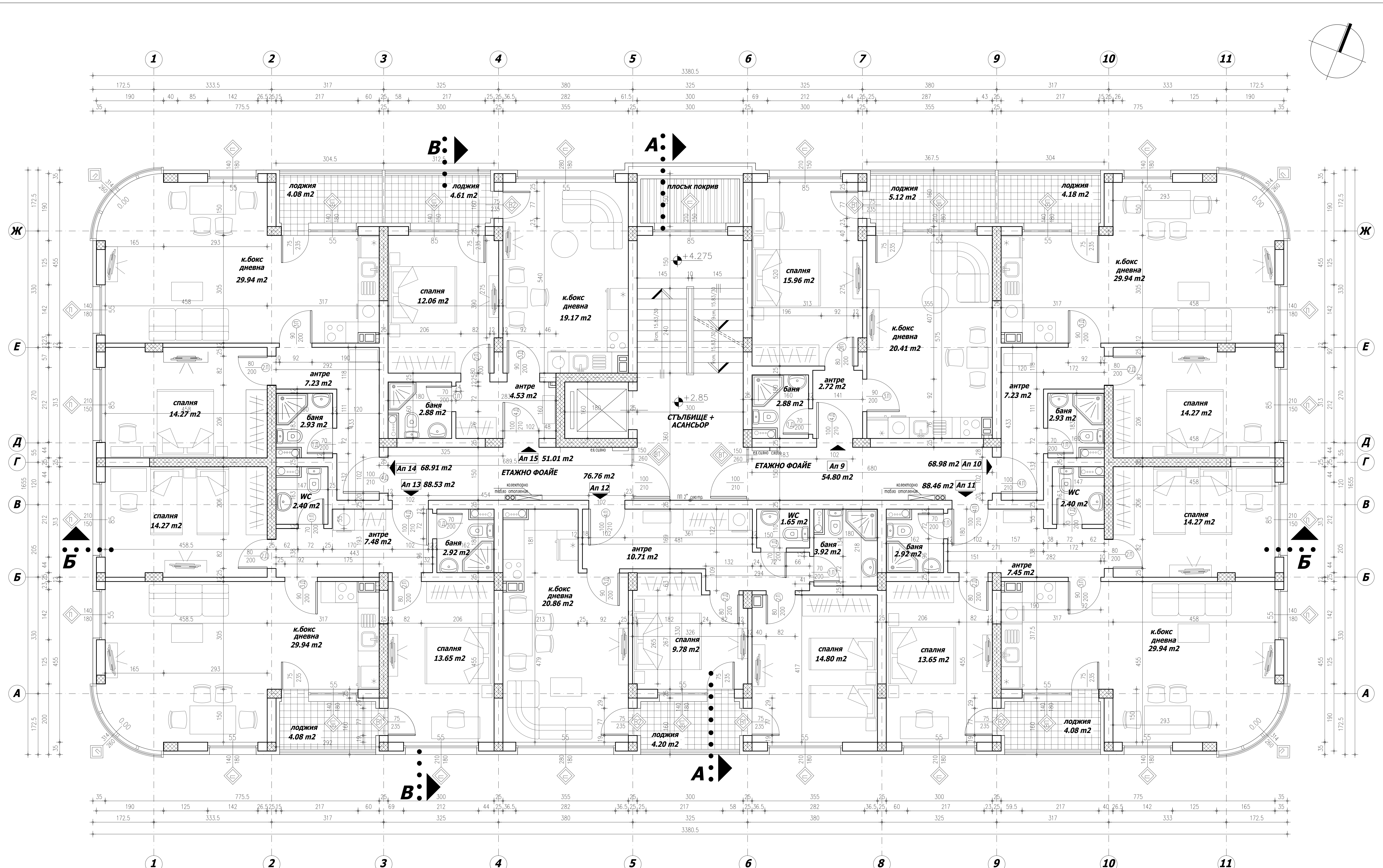
РАЗПРЕДЕЛЕНИЕ ВТОРИ ЕТАЖ М 1:50
