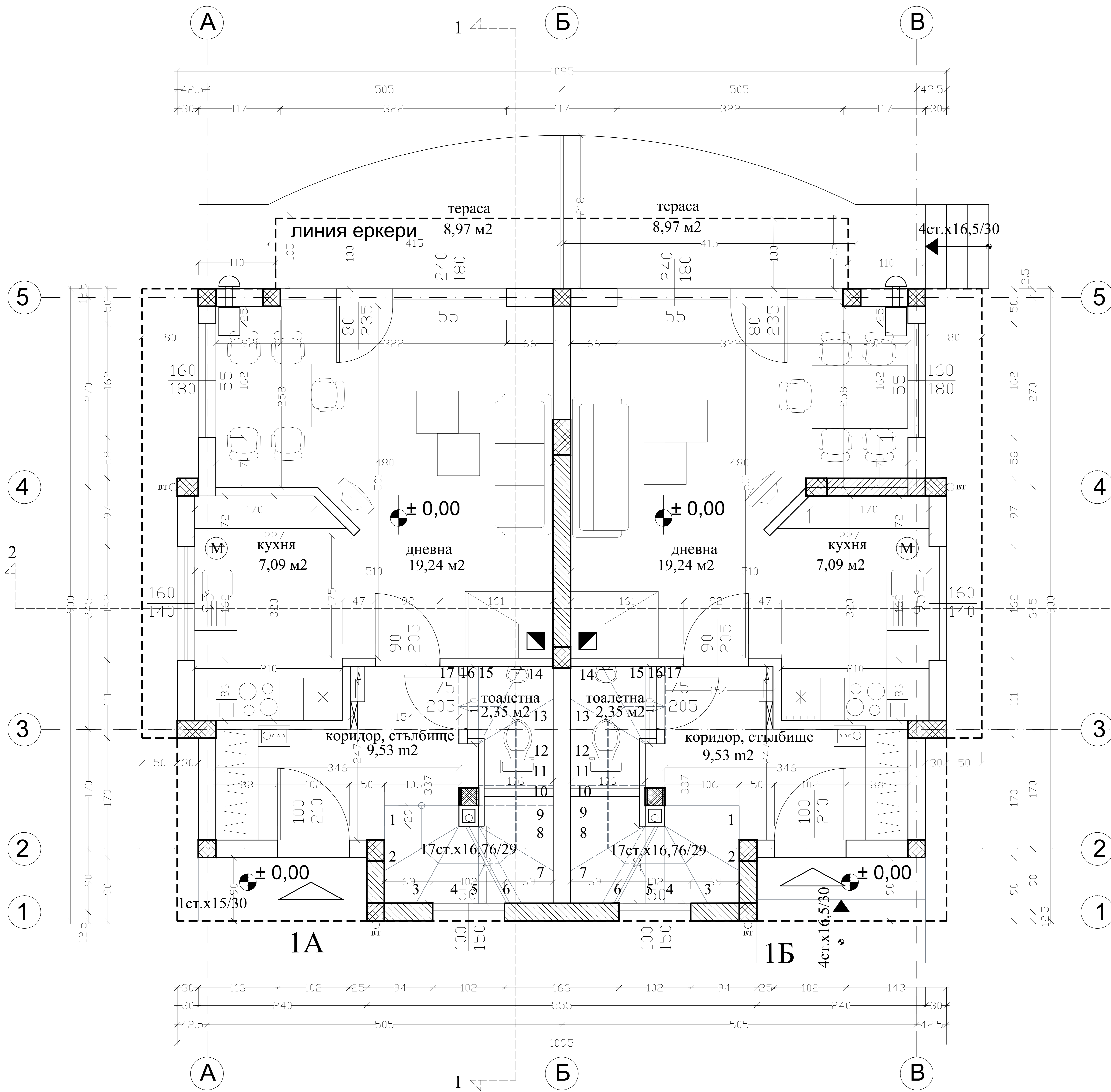
КЪЩА 1 - Кота ±0,00=802,19
