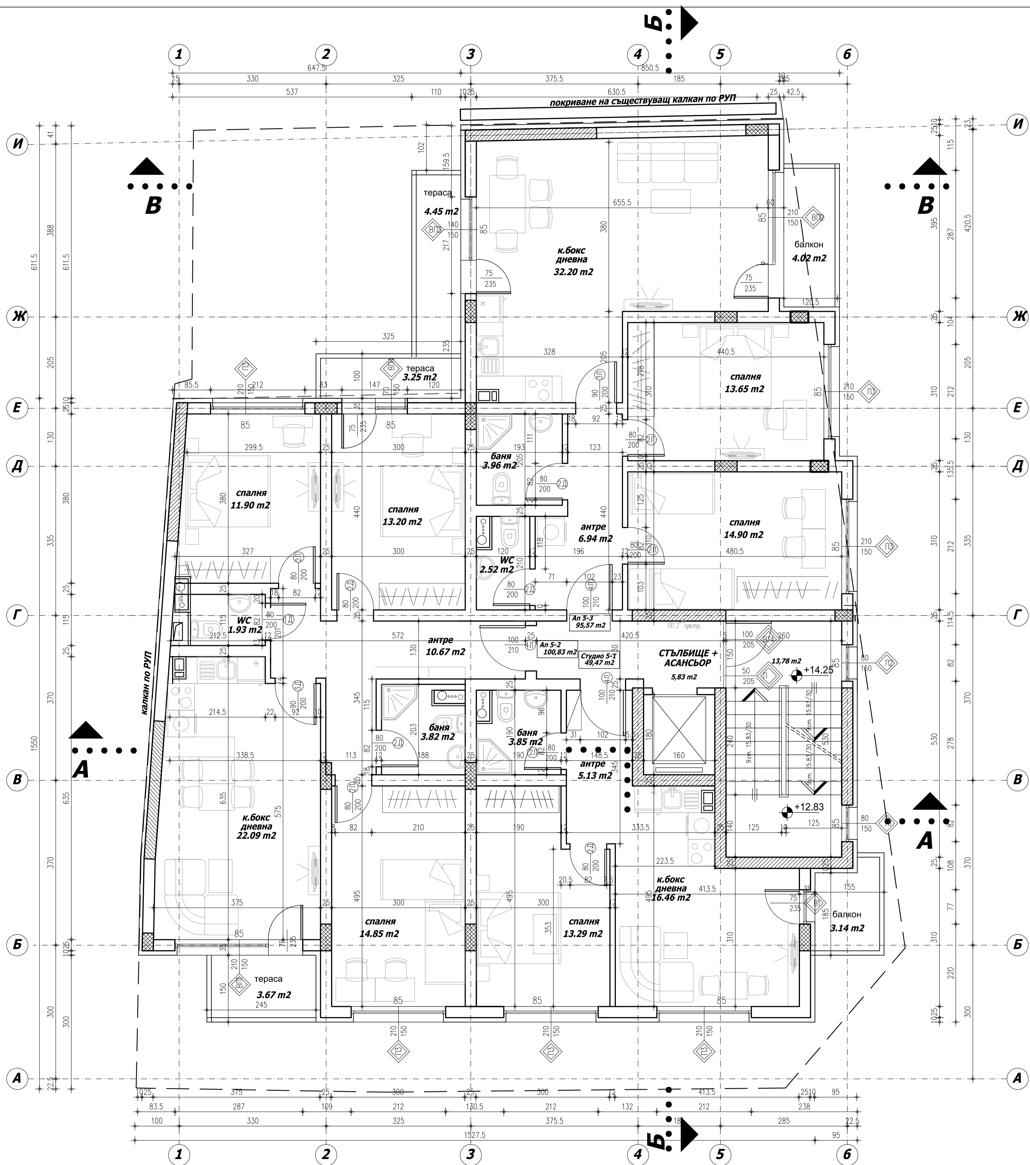
РАЗПРЕДЕЛЕНИЕ V ЖИЛИЩЕН ЕТАЖ М 1:50
