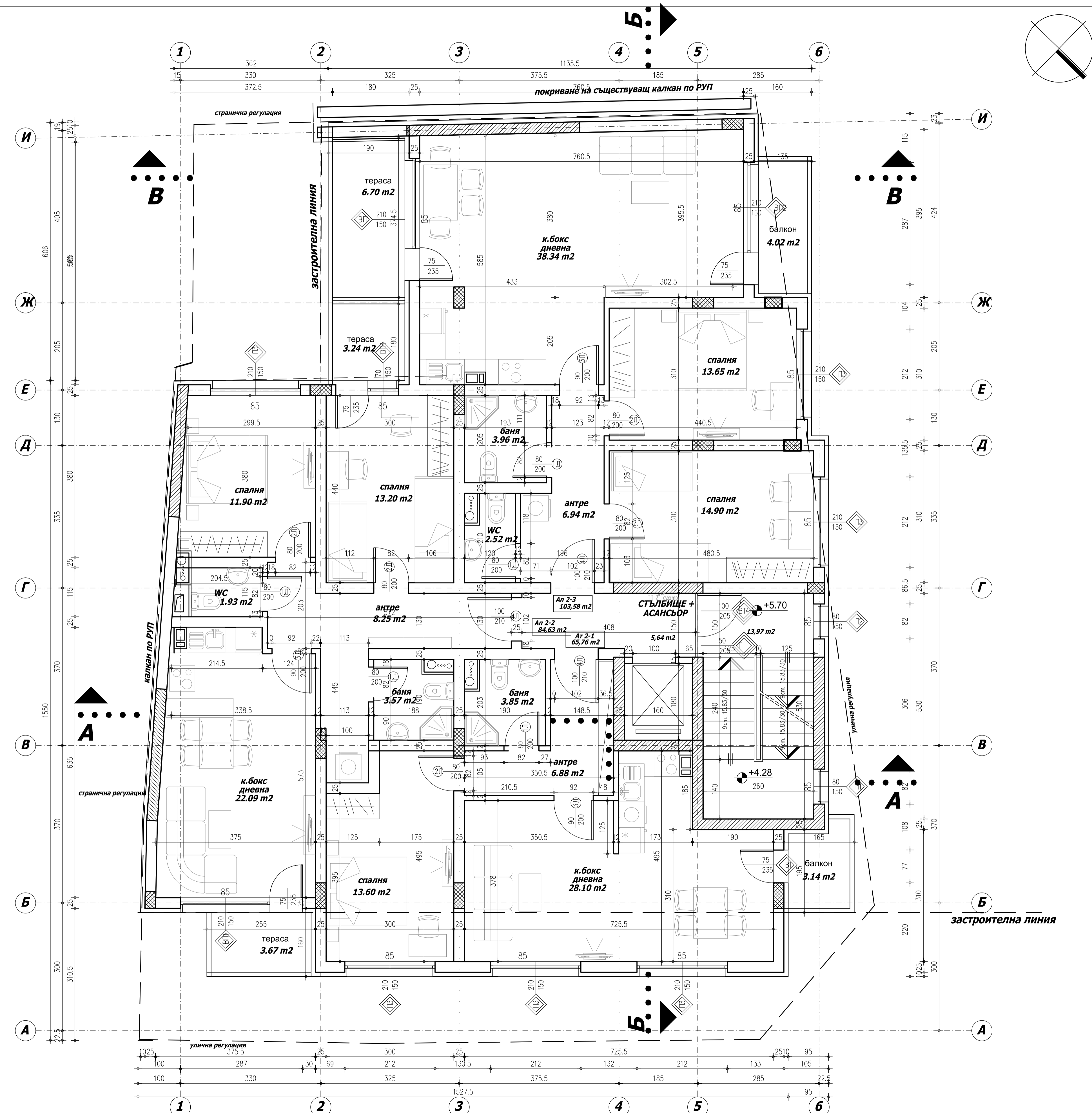
РАЗПРЕДЕЛЕНИЕ II ЖИЛИЩЕН ЕТАЖ М 1:50
