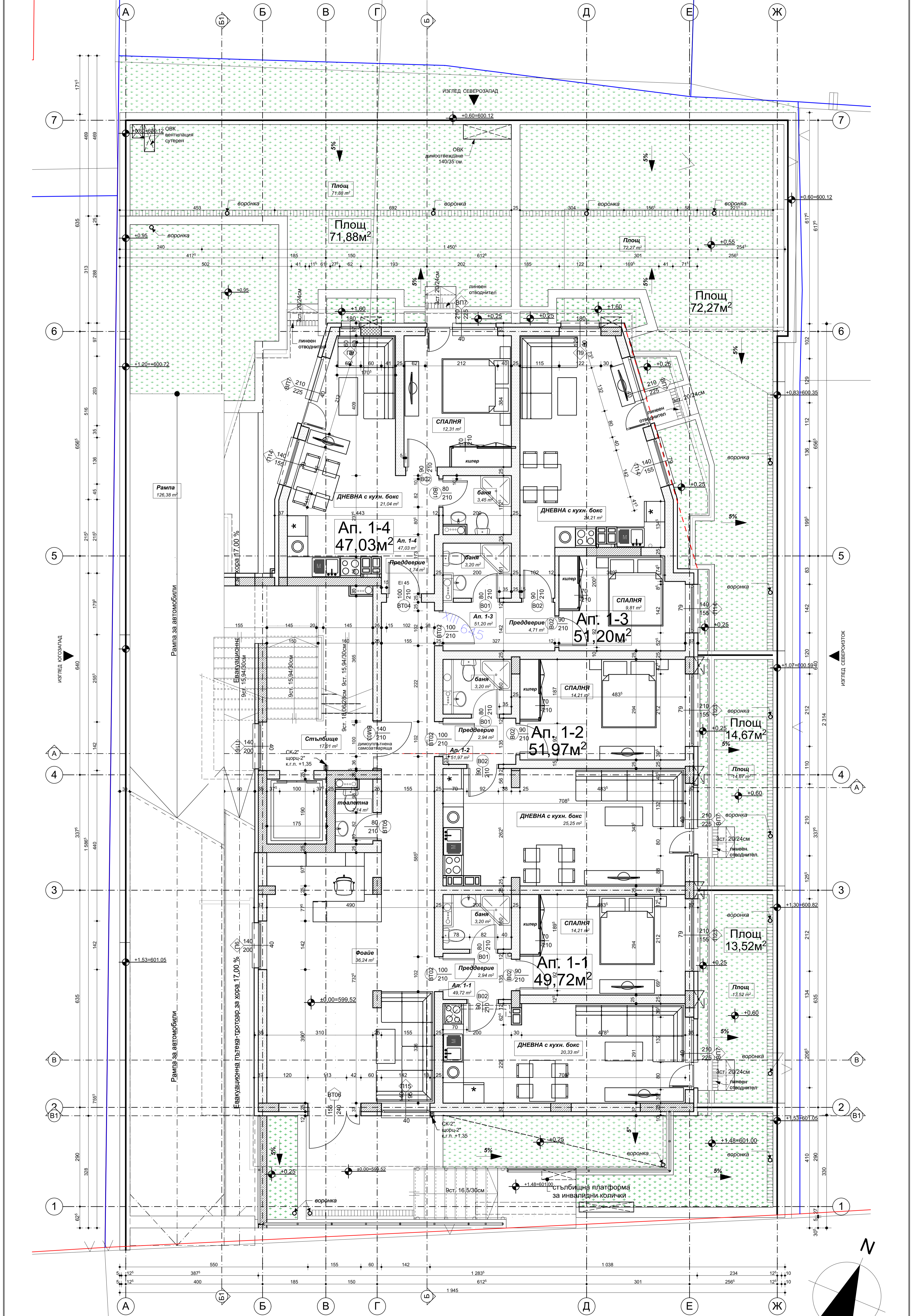
РАЗПРЕДЕЛЕНИЕ ПАРТЕР
