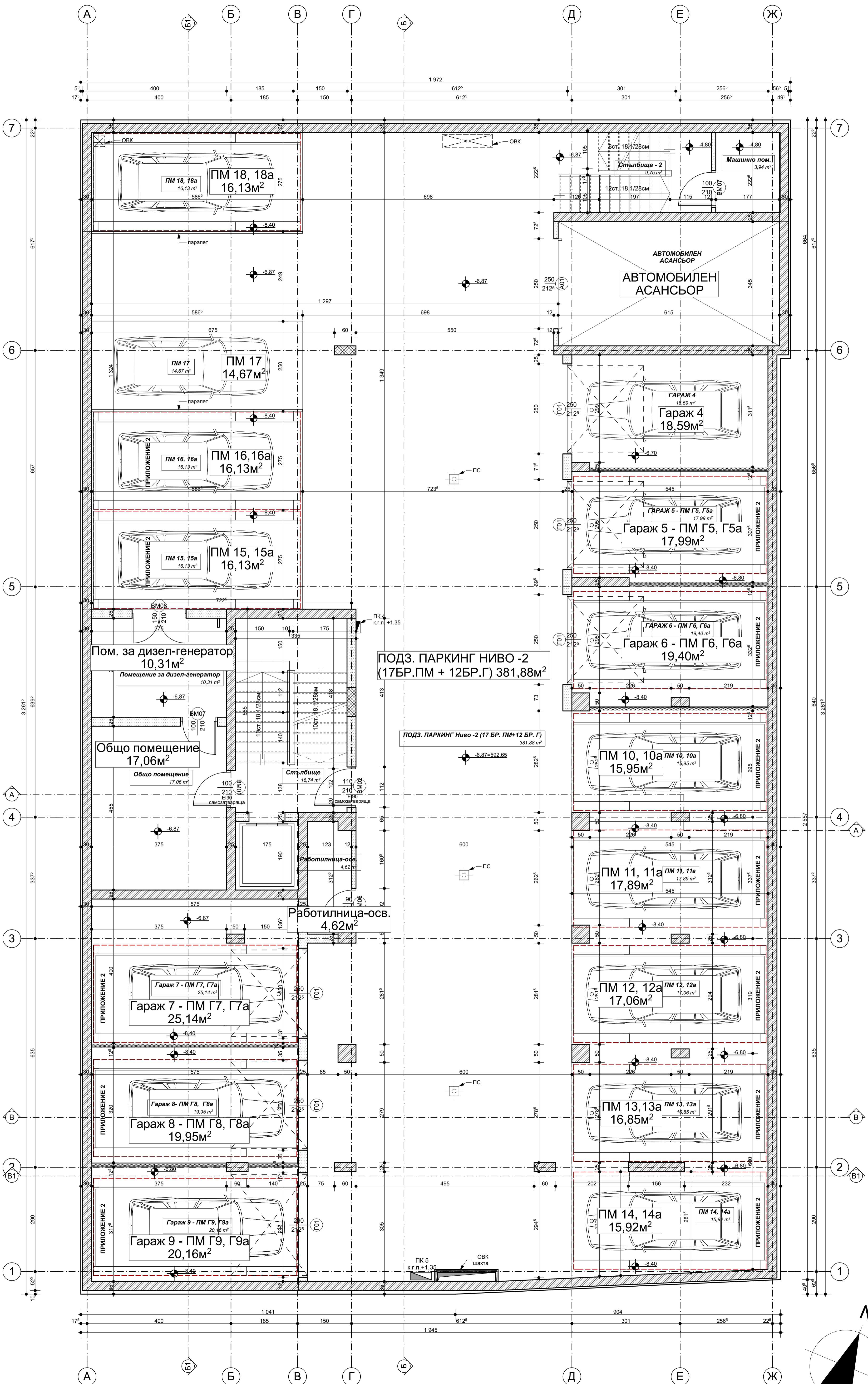
РАЗПРЕДЕЛЕНИЕ ВТОРИ ПОДЗЕМЕН ЕТАЖ
