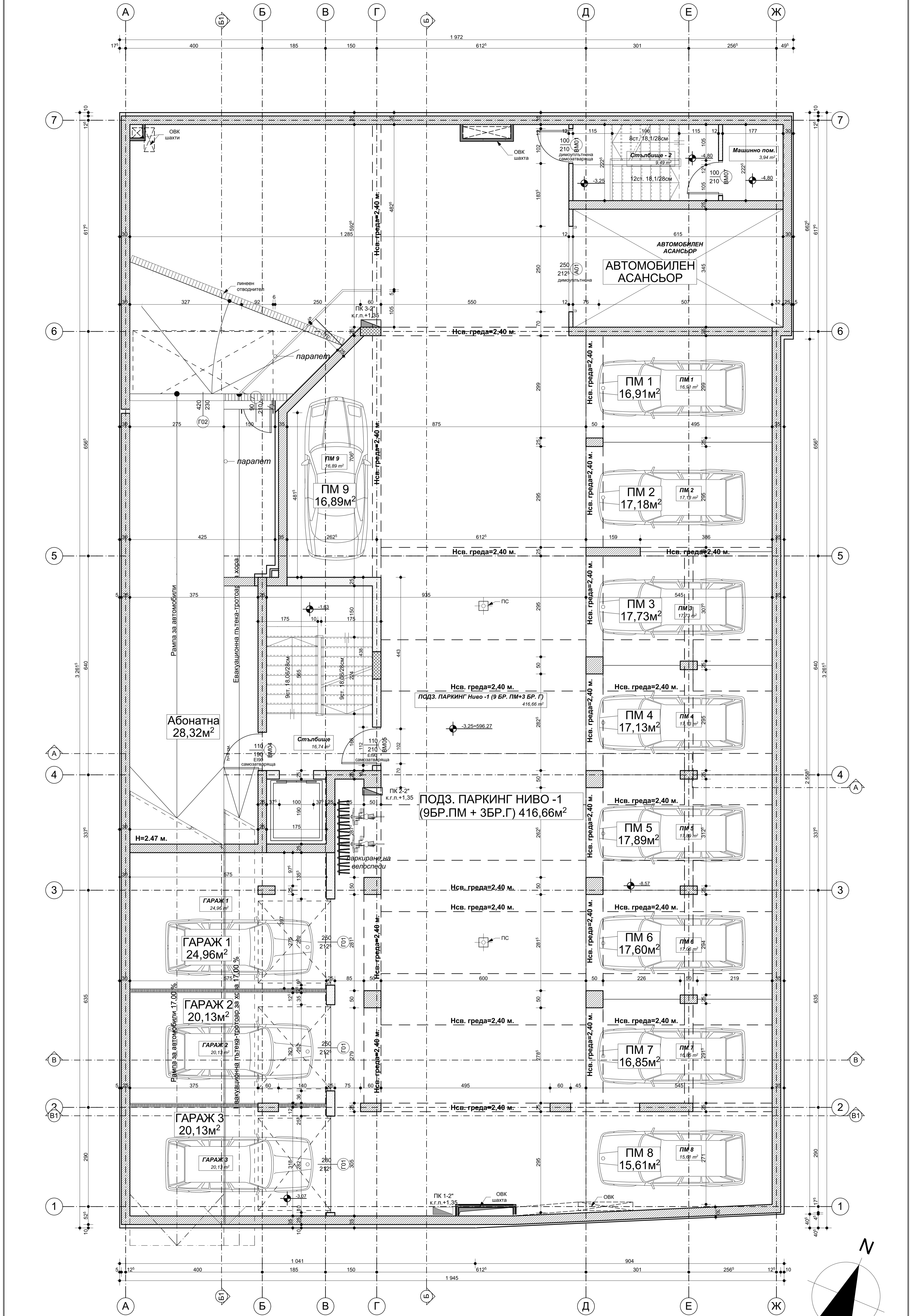
РАЗПРЕДЕЛЕНИЕ ПЪРВИ ПОДЗЕМЕН ЕТАЖ
