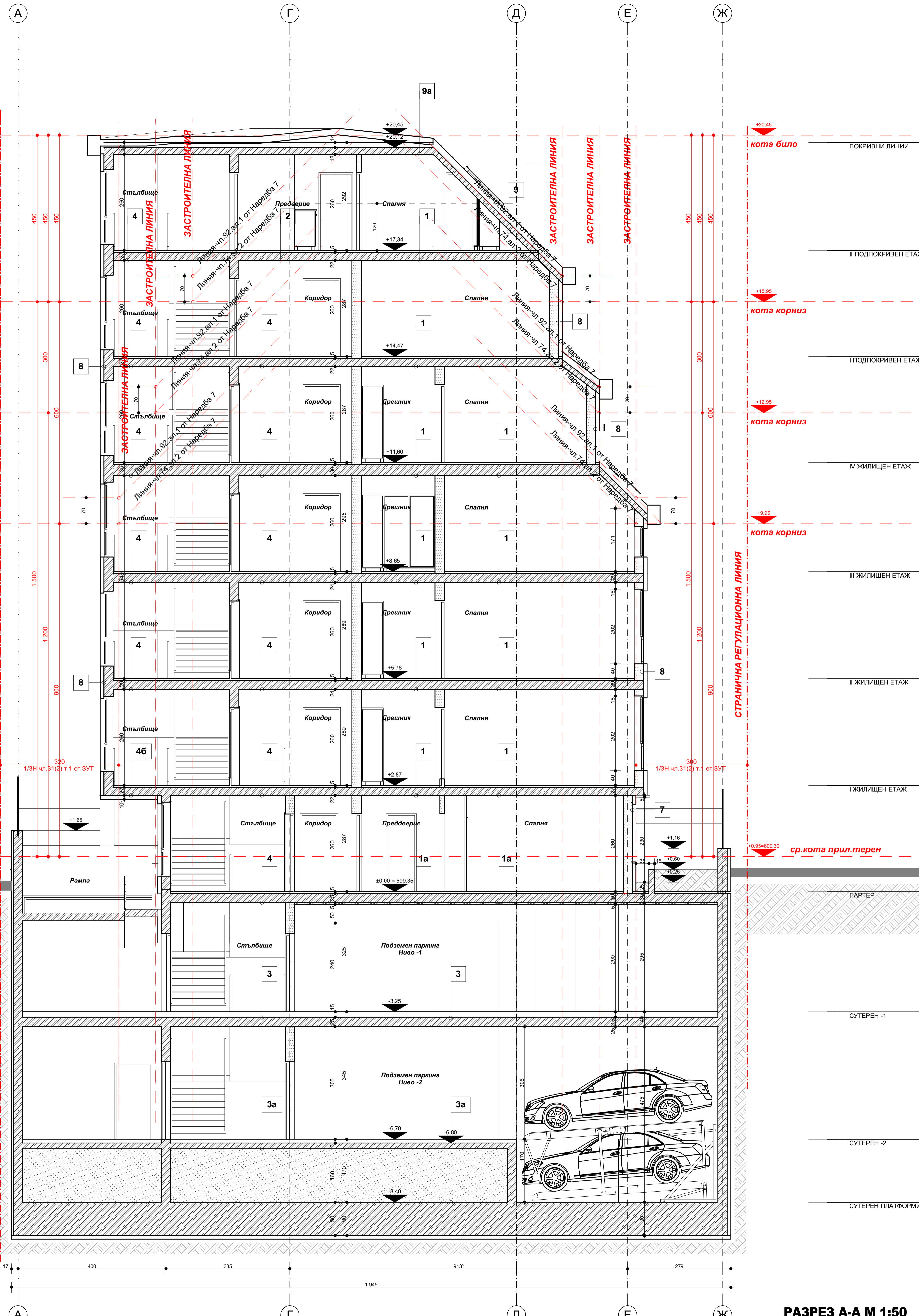
РАЗРЕЗ А-А М 1:50
