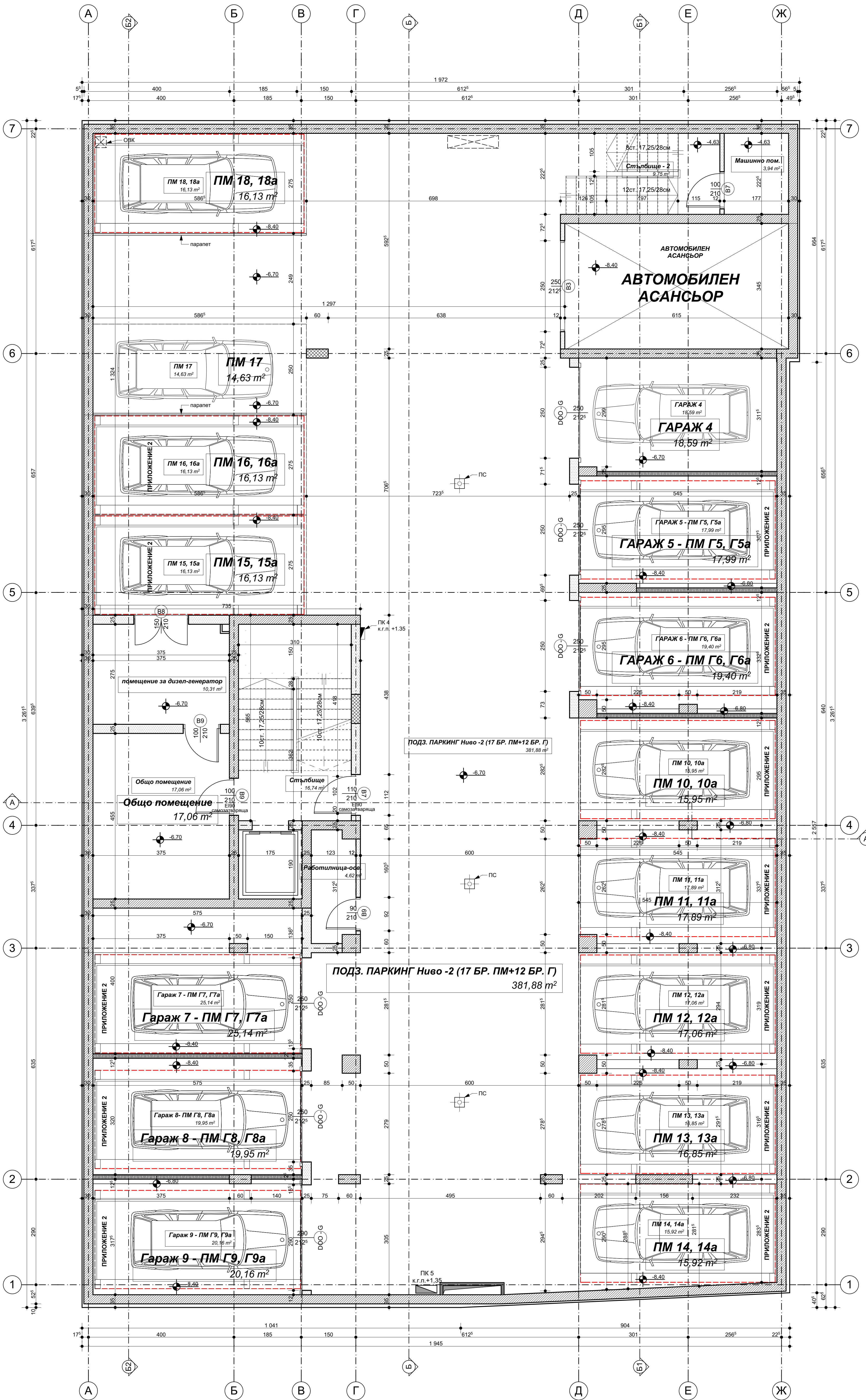
РАЗПРЕДЕЛЕНИЕ СУТЕРЕН КОТА -6,20 М 1:50
