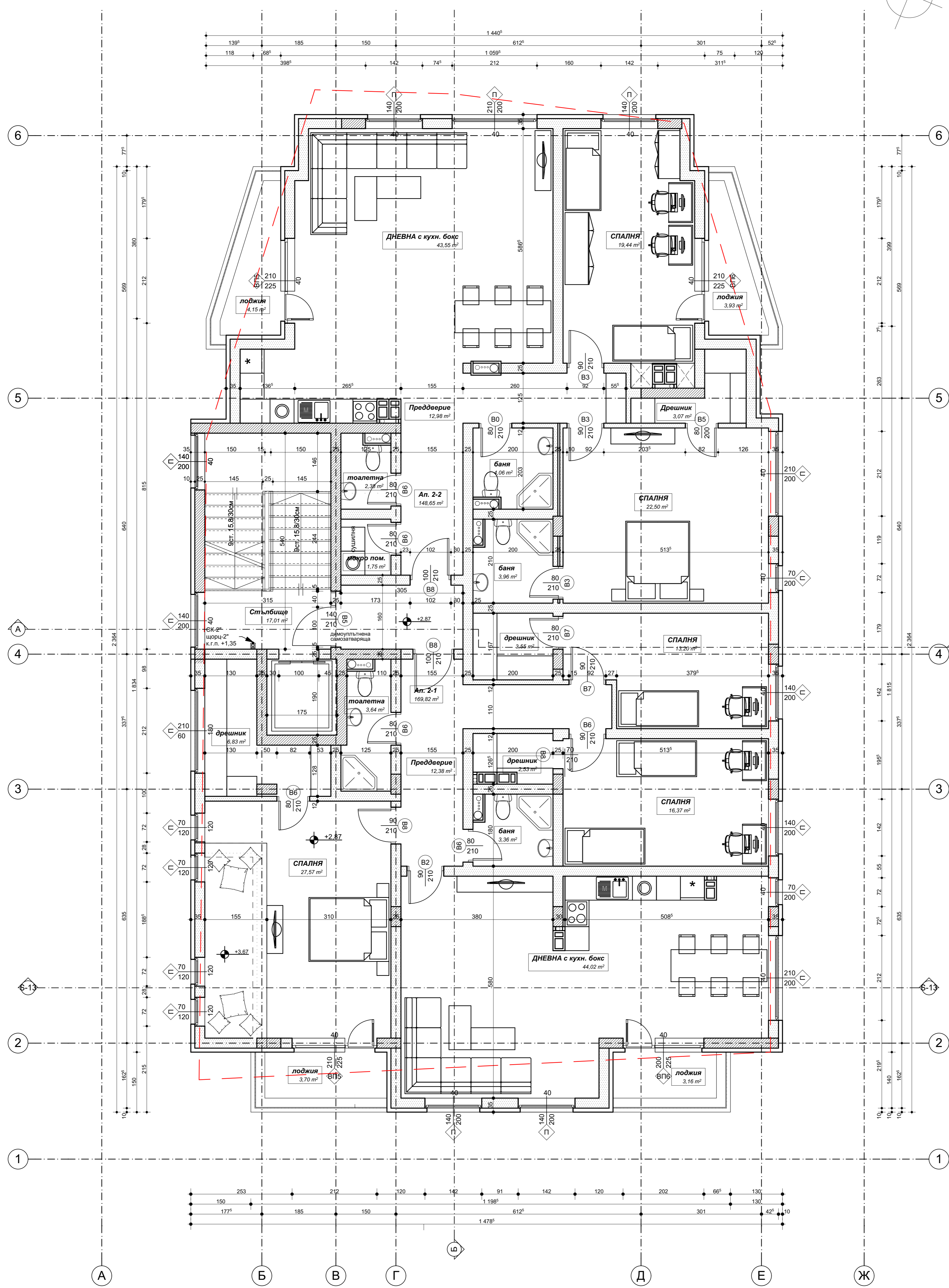
РАЗПРЕДЕЛЕНИЕ КОТА +2,87 М 1:50
