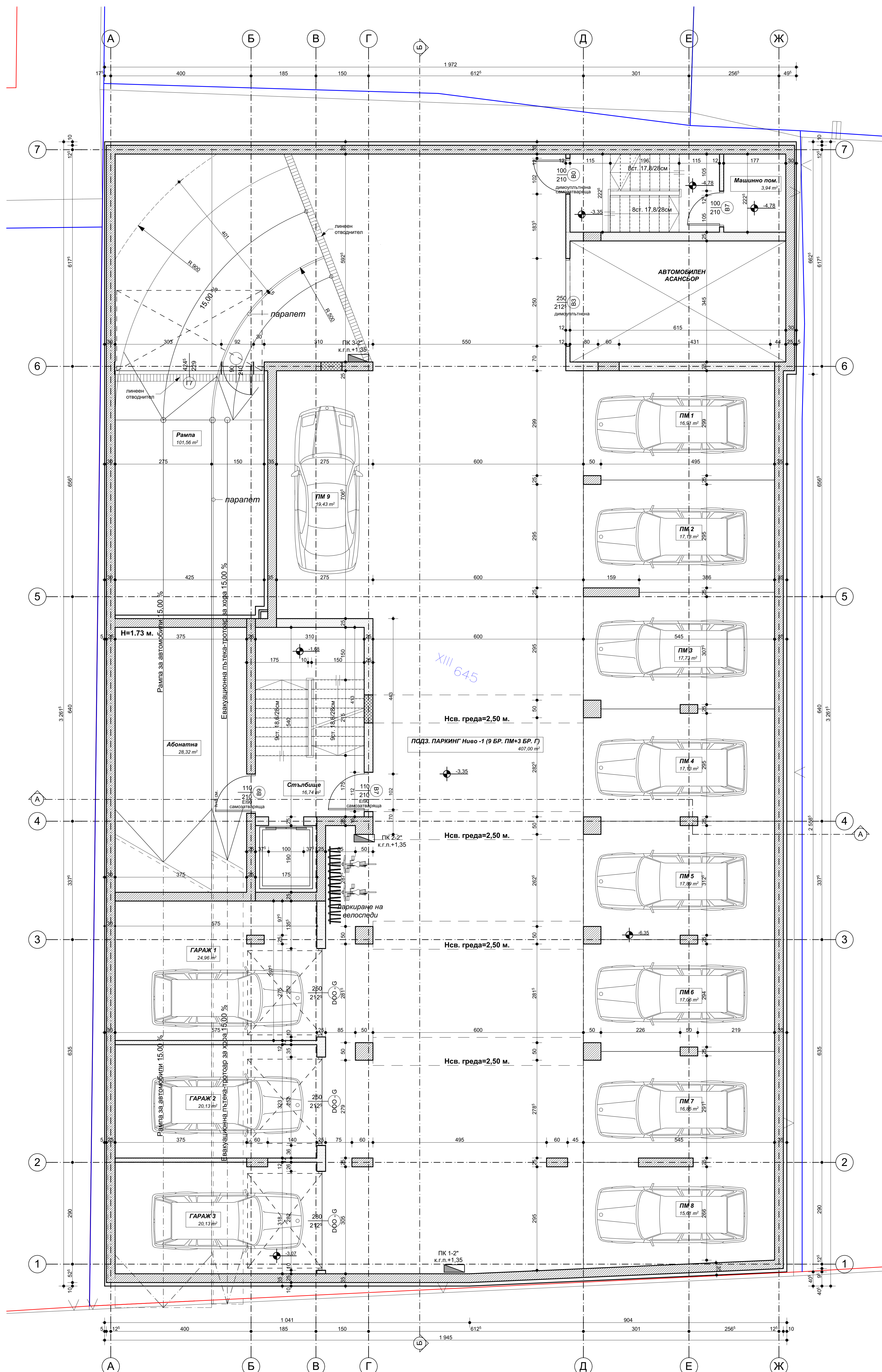
РАЗПРЕДЕЛЕНИЕ СУТЕРЕН КОТА -3,07 М 1:50
